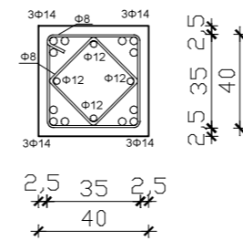
Presjek 1-1 M 1:25
