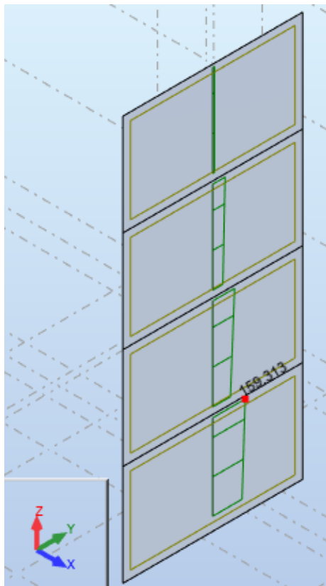
Slika 86. Uzdužna sila F_y
