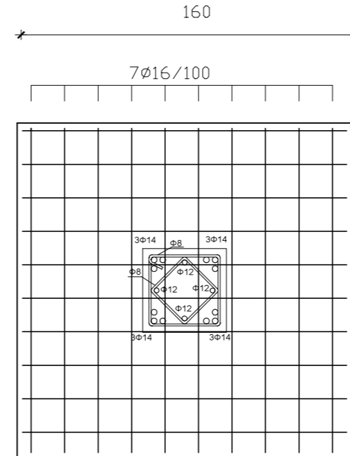
Presjek 2-2 M 1:25
