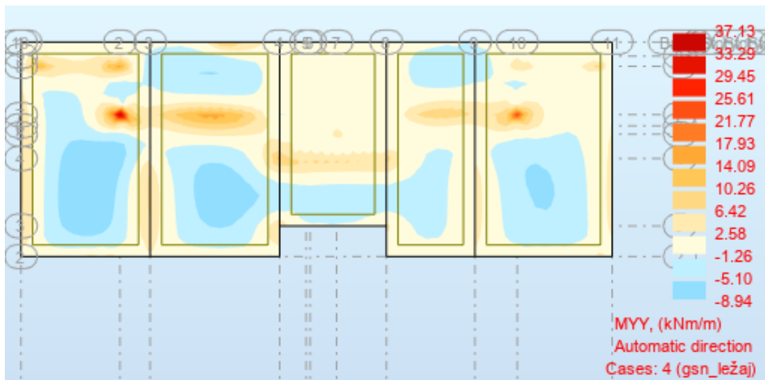
Slika 63. Dijagram momenata savijanja M_{ed,y} (kNm/m)
