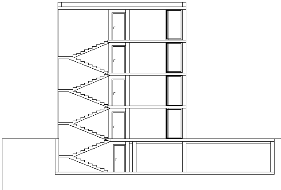
Slika 4. Presjek B-B
