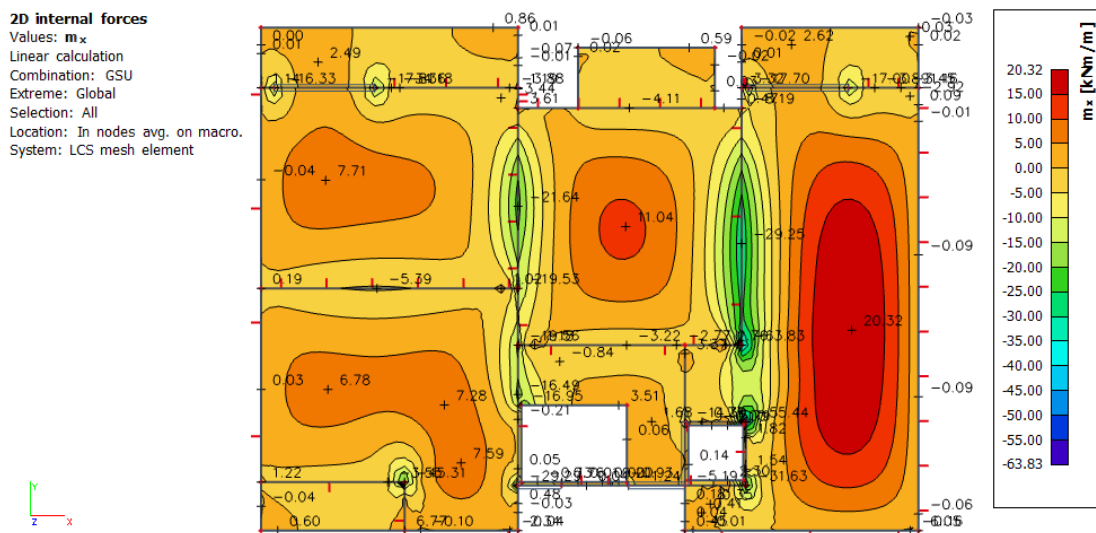
Slika 56. Moment savijanja GSU M_y ploče POZ 200 (kNm)
