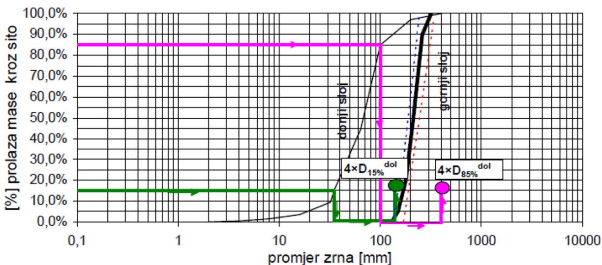
Slika 1.7 Granulometrijska krivulja stijenske mase za izradu lukobrana [2]
