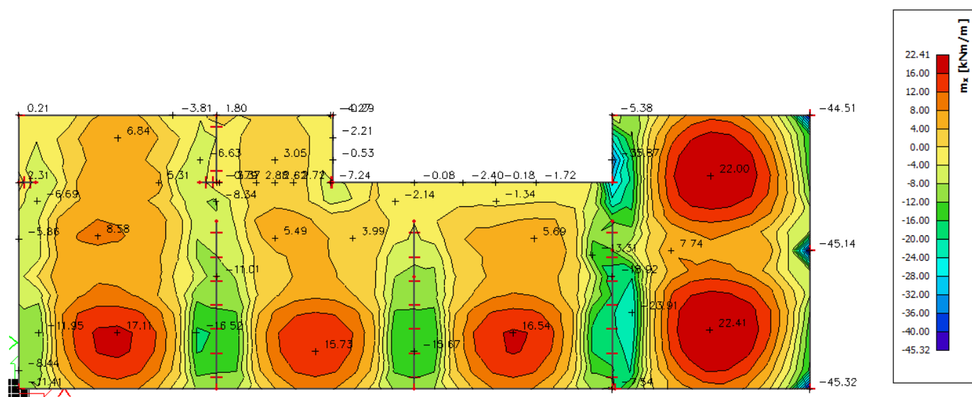
Slika 6.2 Moment savijanja M_{Ed,x} (kNm/m) za GSN-1
