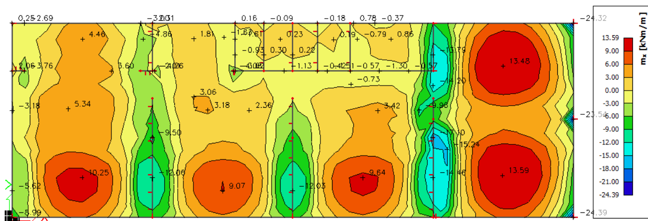
Slika 6.23 Moment savijanja M_{Ed,x} (kNm/m) za GSU-1
