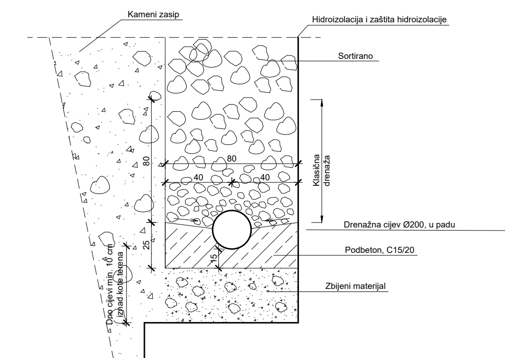
Detalj drenáže
