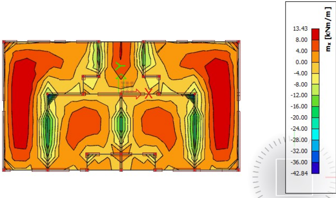
Slika 46 M_{sd,x} [ \text{kNm/m} ] = računski momenti savijanja u smjeru lokalnih osi za q_{sd}=1.35 G + 1.5Q
