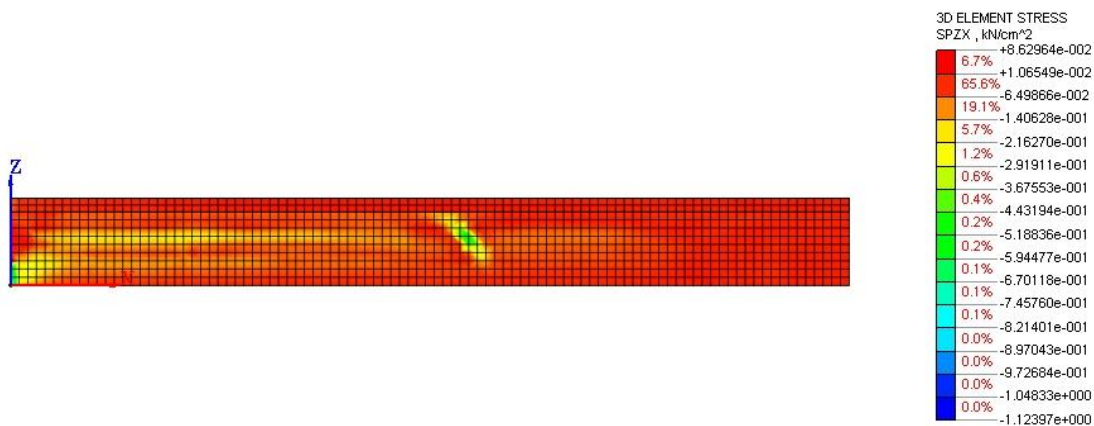
Slika 110: Naprezanja xz (kN/cm 2 )
