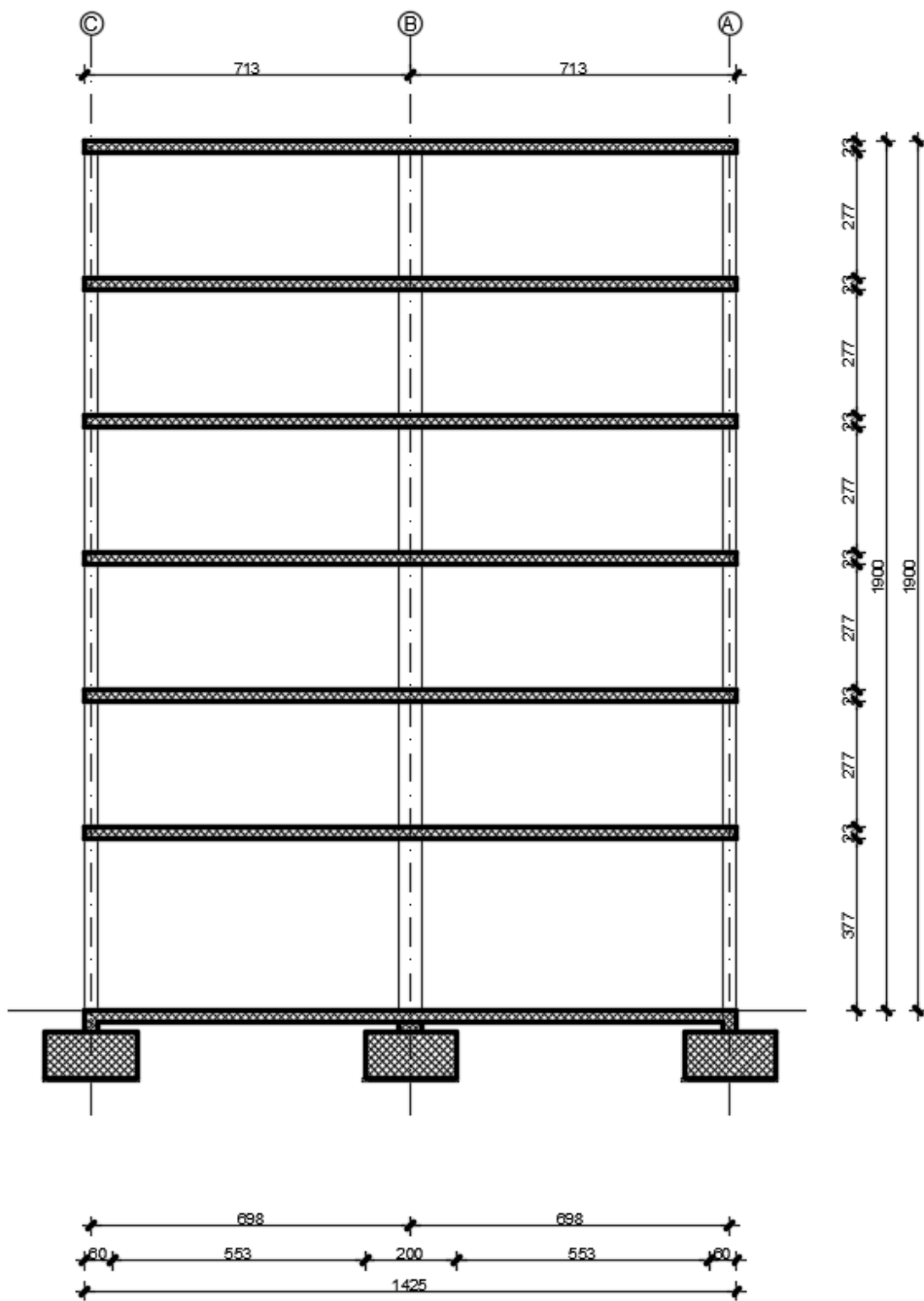
Slika 1.3 Poprečni presjek B-B
