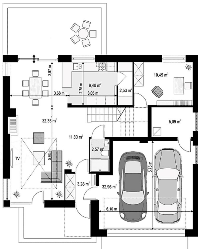
Slika 16. Tlocrt prizemlja
