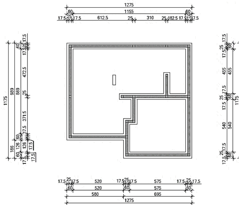
Slika 18. Tlocrt temelja
