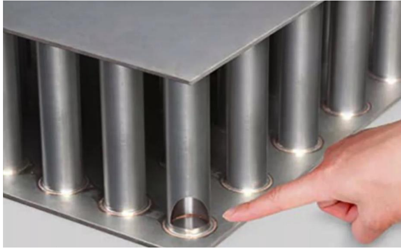
Slika 12. B-Core ploča
