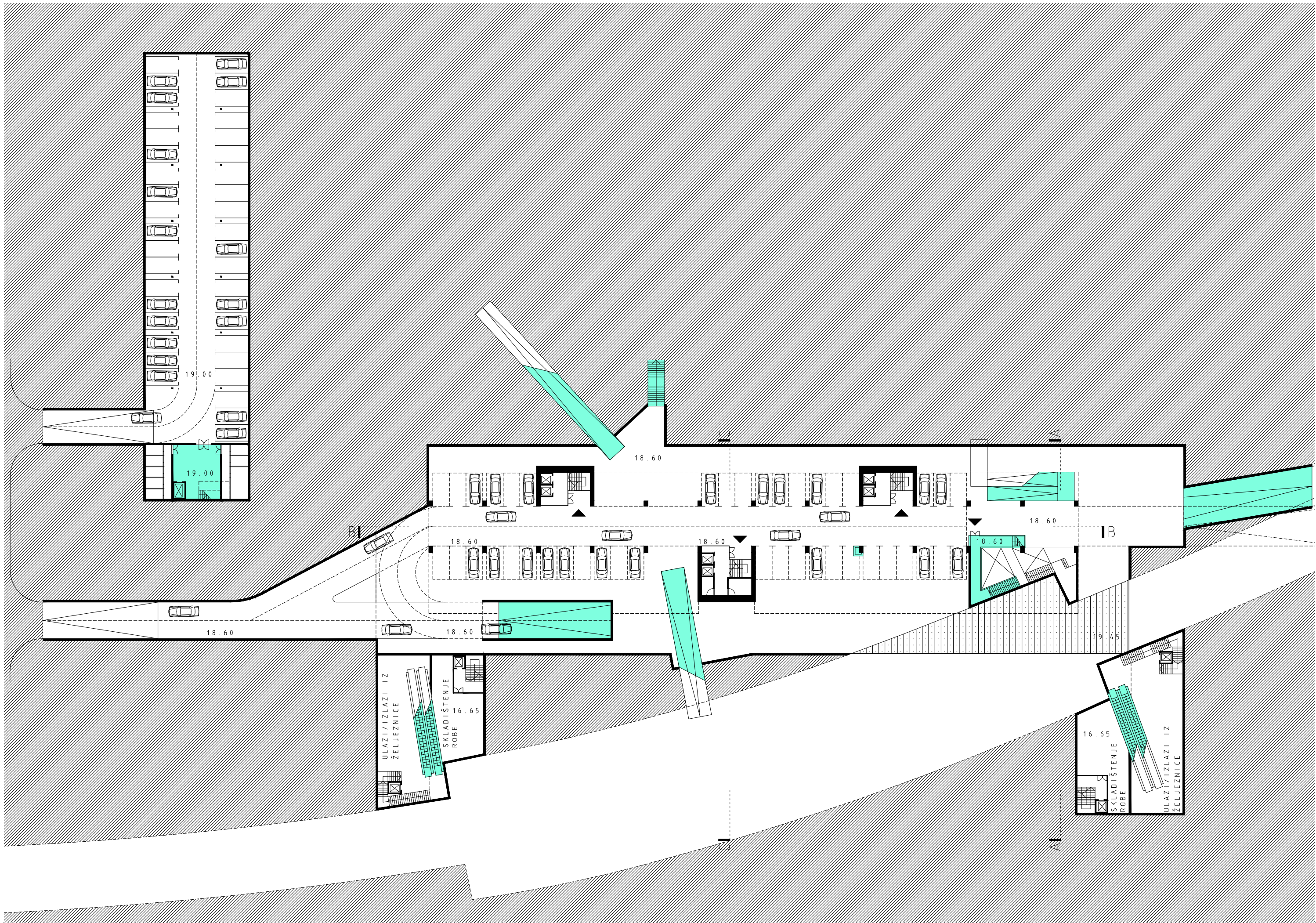
0 5 20 M 1:500 tlocrt razina 0
