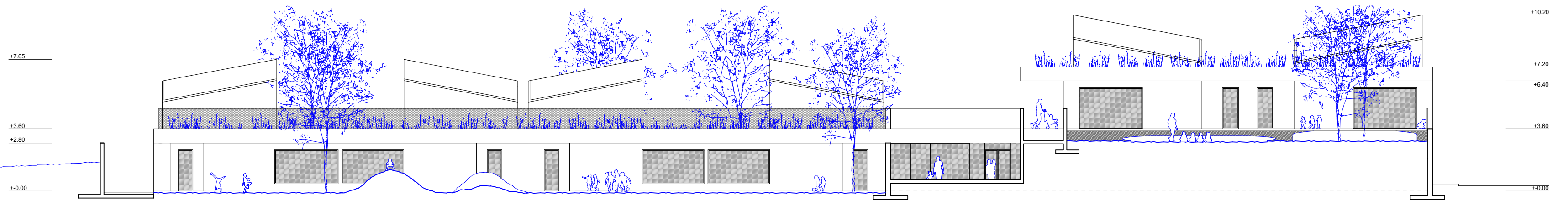
JUŽNO PROČELJE
