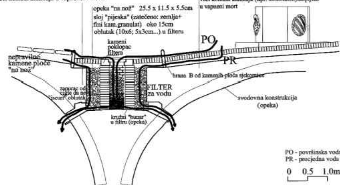
Shema filtriranja vode
