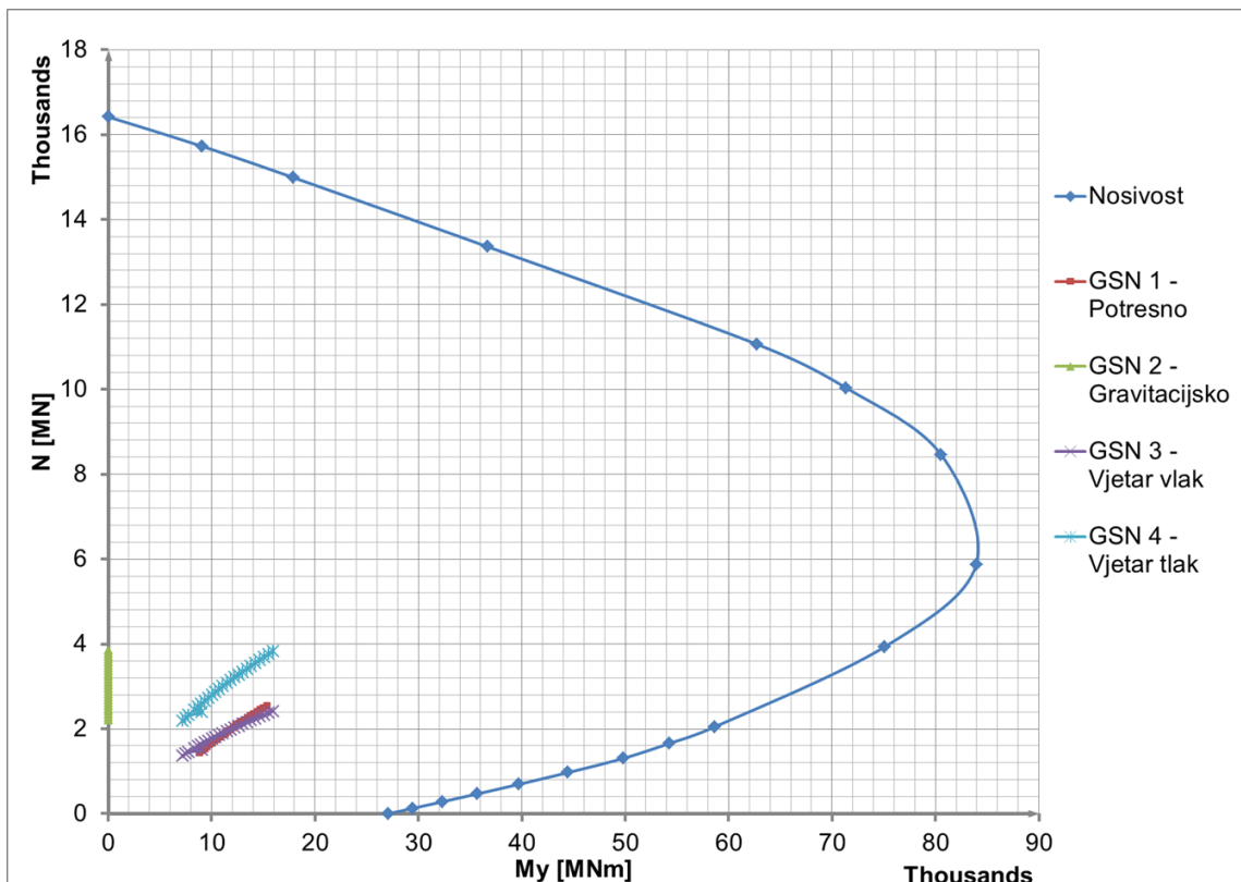
Slika 7.4.3.6 Dijagram nosivosti za presjek 700-800 m
