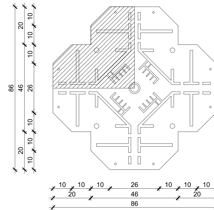
SHEMA TLOCRTA - RAZINA 300-500 m M 1:1000
