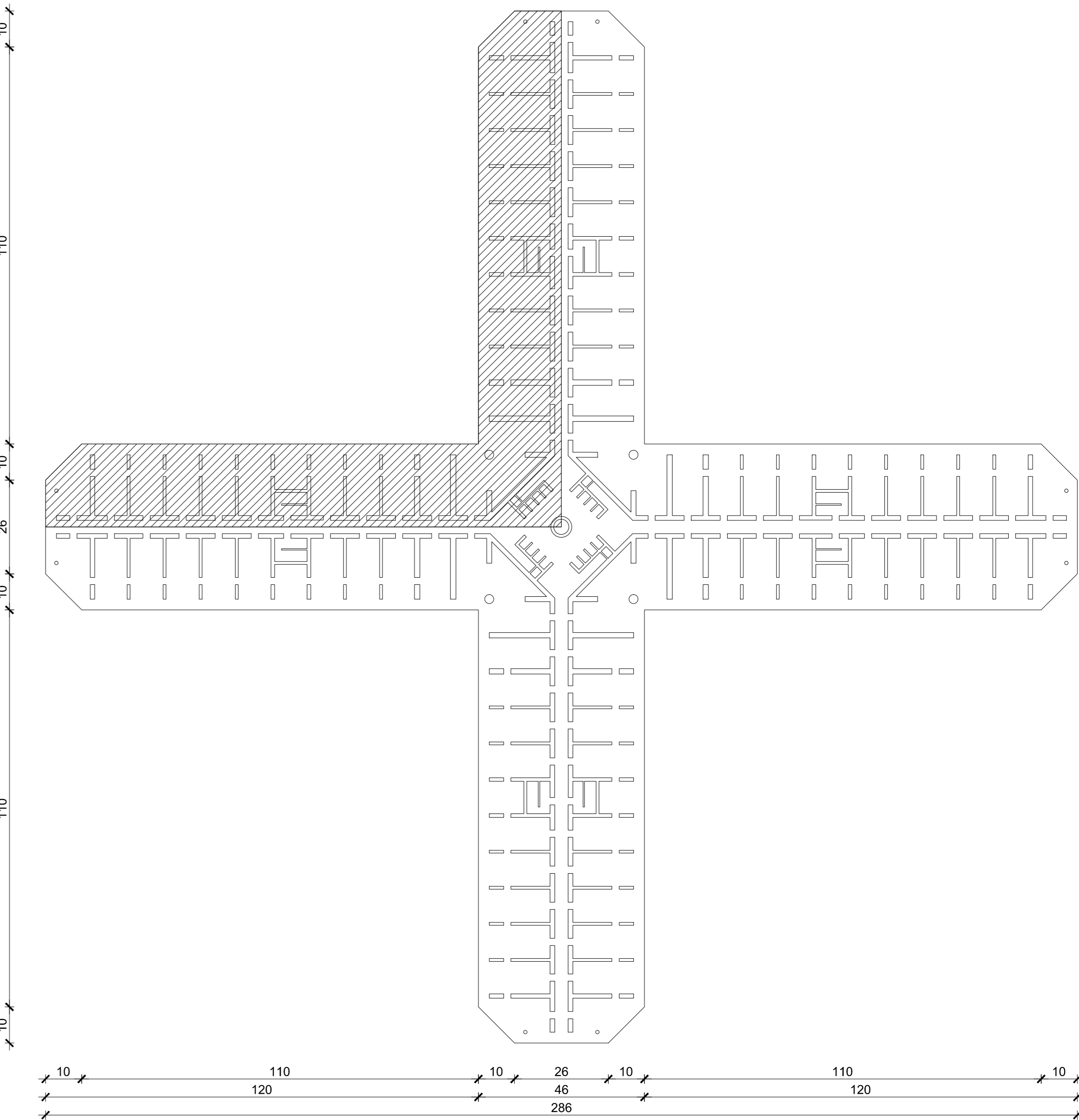
HEMA TLOCRTA - RAZINA 0-52 m M 1:1000
