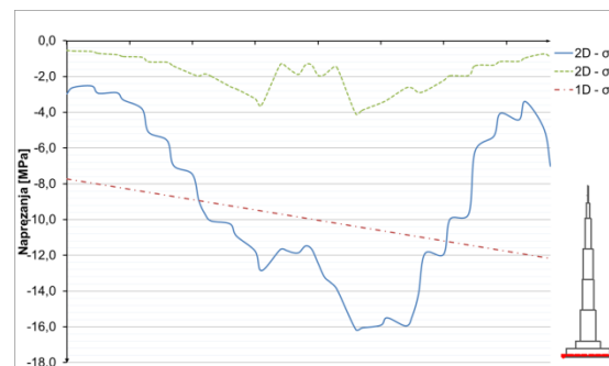
Slika 8.1.3.4 Naprezanja u betonu u presjeku h=0 m – opterećenje vjetrom
