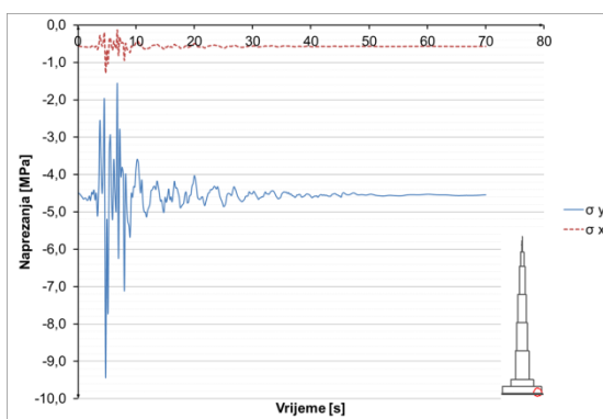
Slika 8.3.5.17 Naprezanja u betonu u presjeku h=0 m – potres Bingöl
