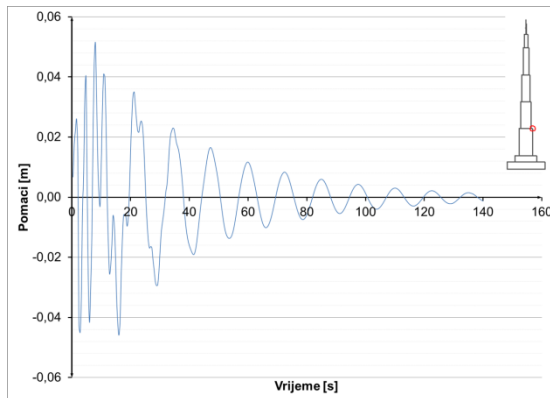
Slika 8.3.3.10 Pomaci u presjeku h=300 m – potres Banja Luka
