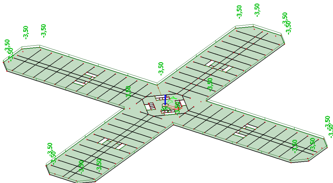
Slika 6.1.2.2 Korisno opterećenje
