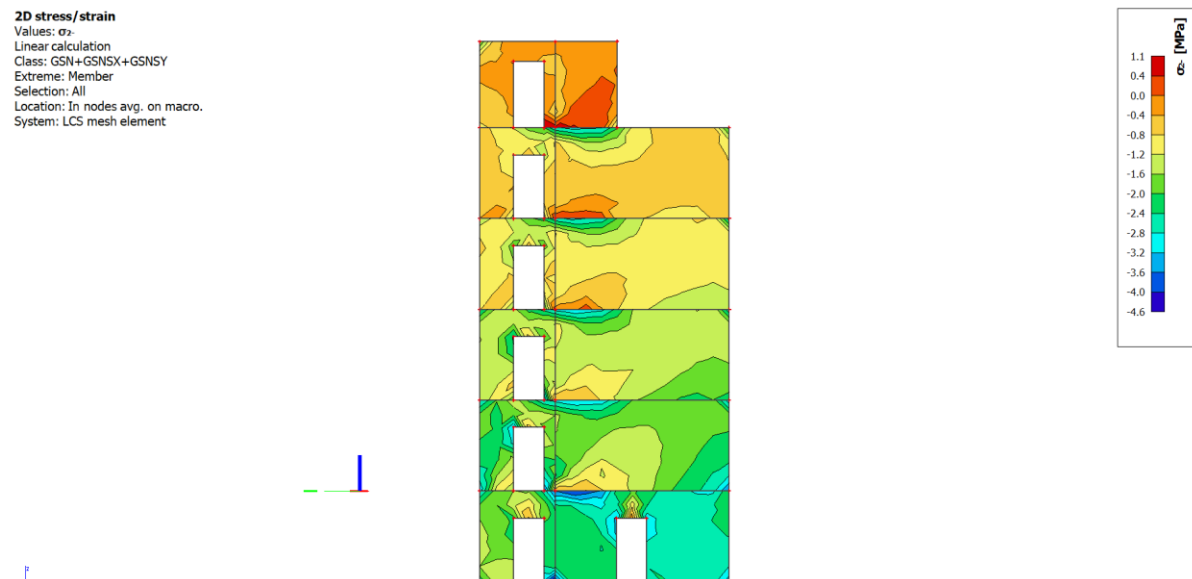
Slika 9.1.24. Naprezanja \sigma_2 za anvelopu opterećenja (GSNSX+GSNSY+GSN)
