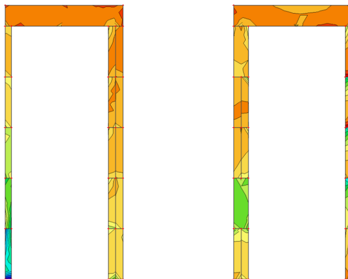
Slika 9.1.14. Naprezanja \sigma_2 za anvelopu opterećenja (GSNSX+GSNSY+GSN)
