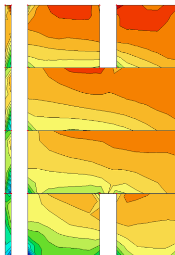
Slika 9.1.45. Naprezanja \sigma_2 za anvelopu opterećenja (GSNSX+GSNSY+GSN)
