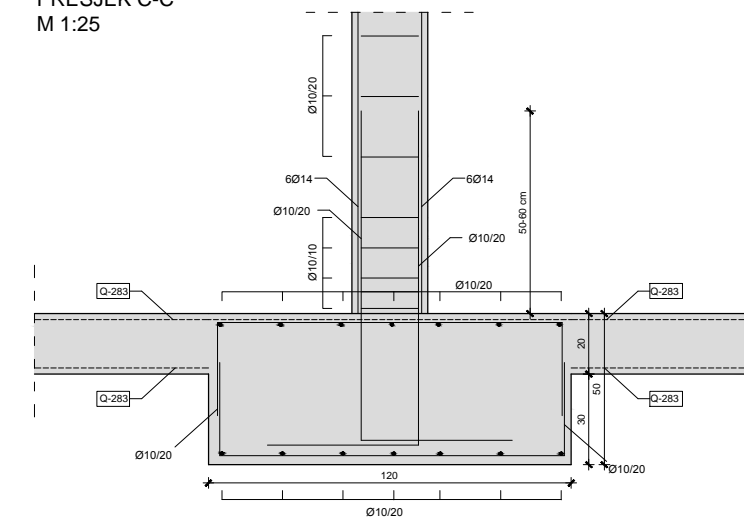
PRESJEK C-C M 1:25
