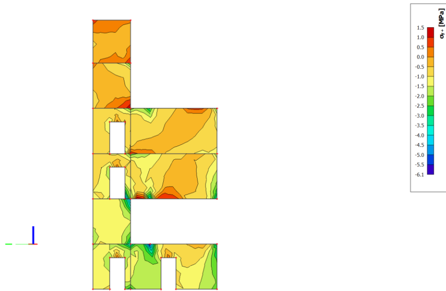
Slika 9.1.37. Naprezanja \sigma_y za anvelopu opterećenja (GSNSX+GSNSY+GSN)
