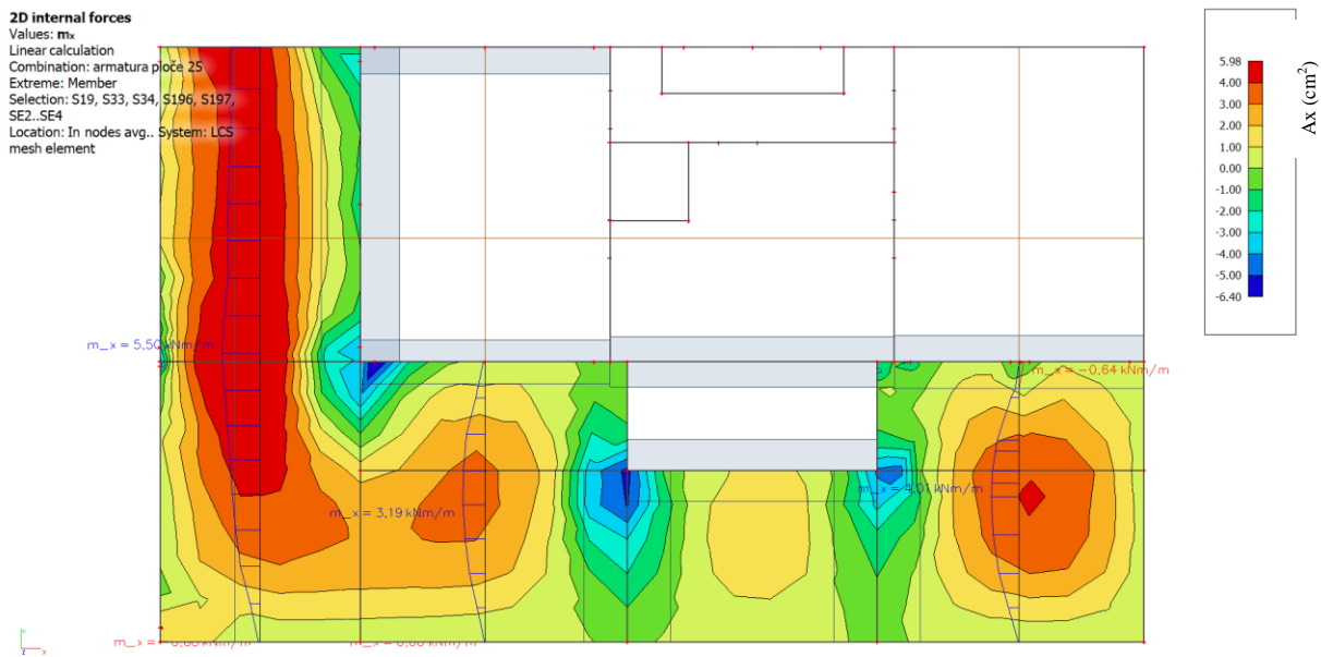
Slika 8.1.7. Armatura ploče d=25\text{cm} smjer x-x za GSN
