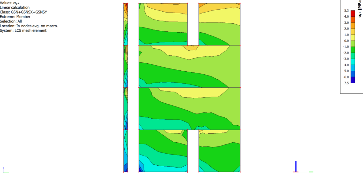
Slika 9.1.43. Naprezanja \sigma_y za anvelopu opterećenja (GSNSX+GSNSY+GSN)
