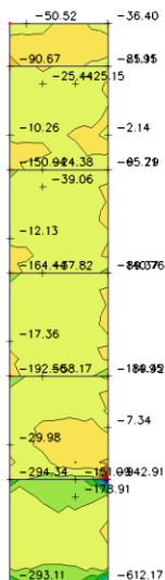
Slika 9.1.30. Uzdužna sila nx za anvelopu opterećenja (GSNSX+GSNSY+GSN)
