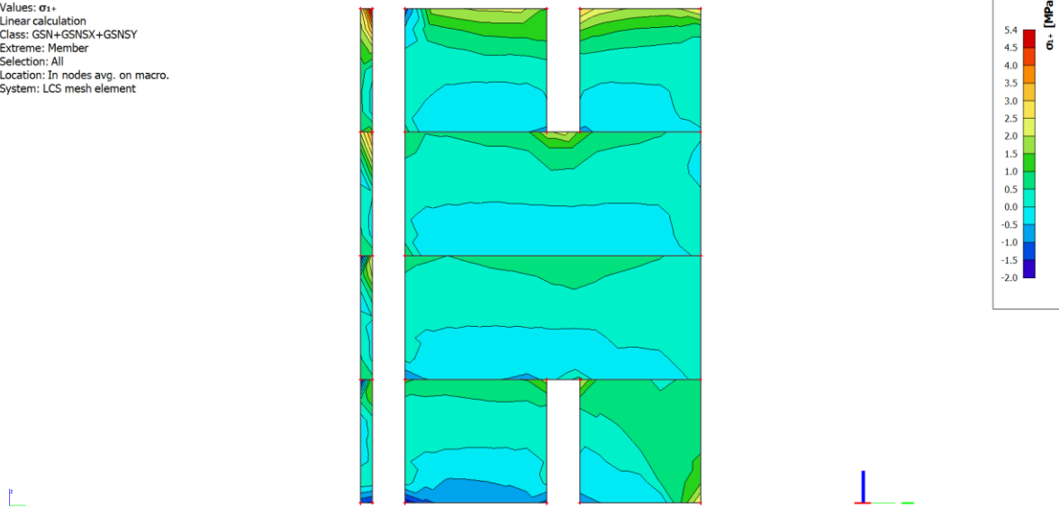
Slika 9.1.44. Naprezanja \sigma_1 za anvelopu opterećenja (GSNSX+GSNSY+GSN)
