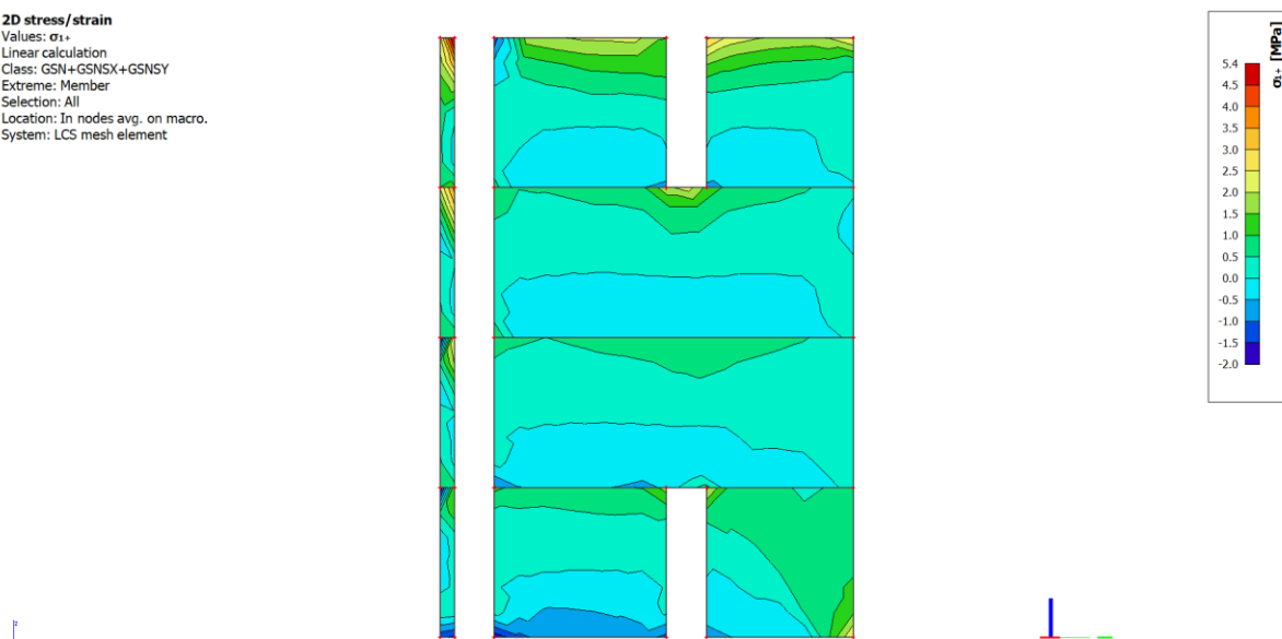
Slika 9.1.44. Naprezanja \sigma_1 za anvelopu opterećenja (GSNSX+GSNSY+GSN)
