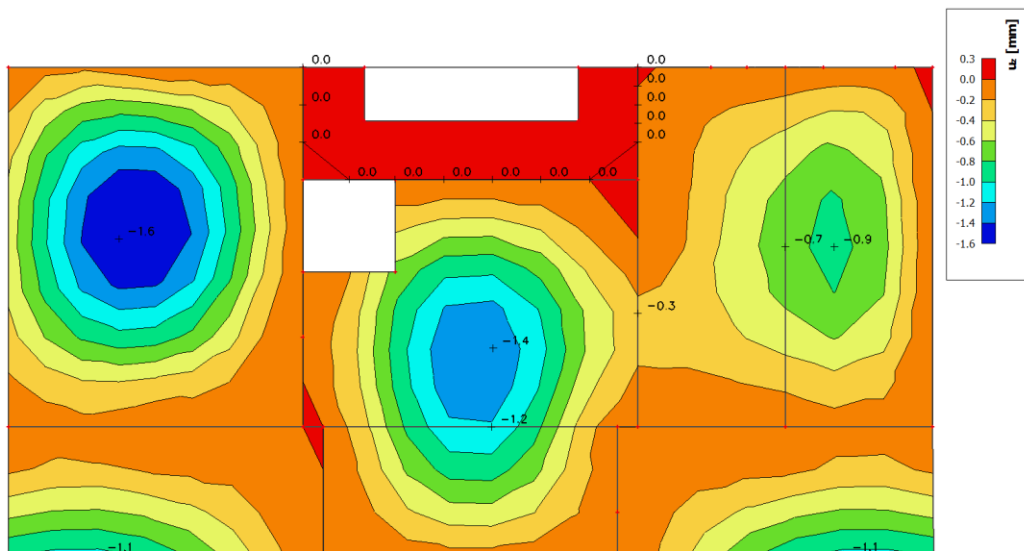
Slika 8.1.27. Progibi ploĉa [mm] za GSU-1 ( \delta EL \leq L/250 )
