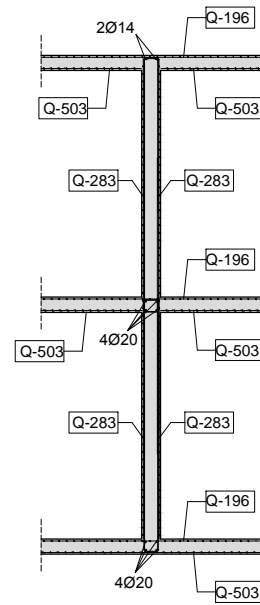
PRESJEK 1-1
