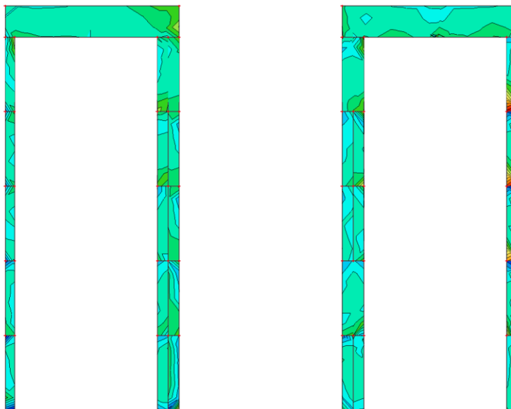
Slika 9.1.13. Naprezanja \sigma_1 za anvelopu opterećenja (GSNSX+GSNSY+GSN)
