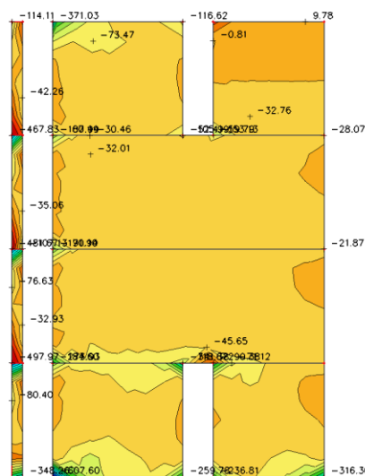
Slika 9.1.44. Uzdužna sila n_x za anvelopu opterećenja (GSNSX+GSNSY+GSN)
