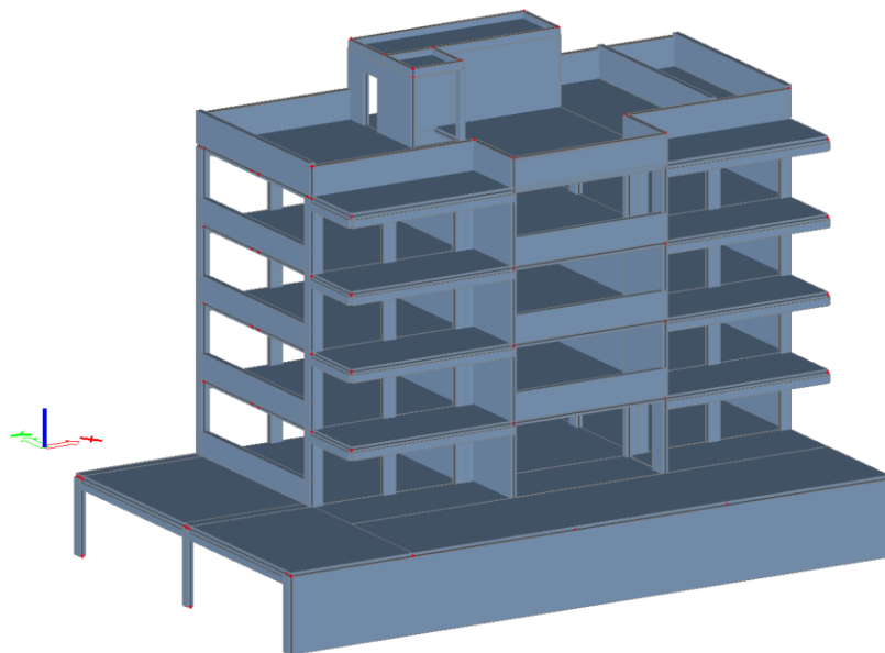
Slika 5.1. Renderirani prikaz modela zgrade - aksonometrija I
