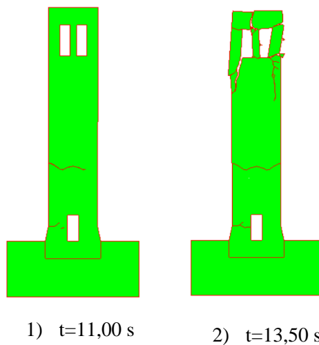
Slika 20. Prikaz nastanka i širenja pukotina pri vršnom ubrzanju tla 5.50g
