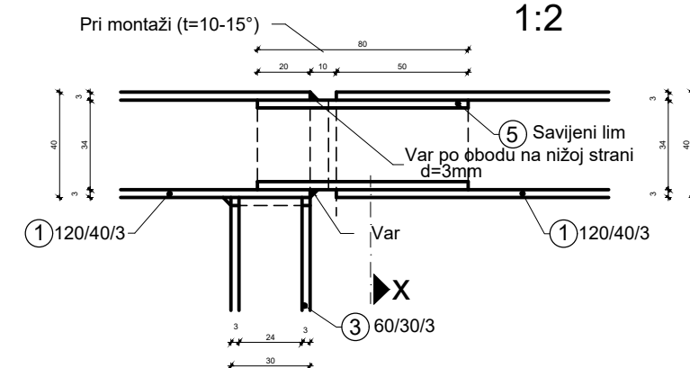
Detalj D 1 1:2
