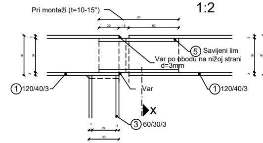
Detalj D 1 1:2
