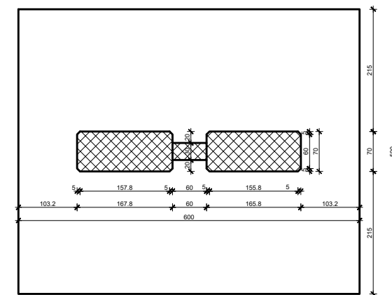
Presjek 4-4
