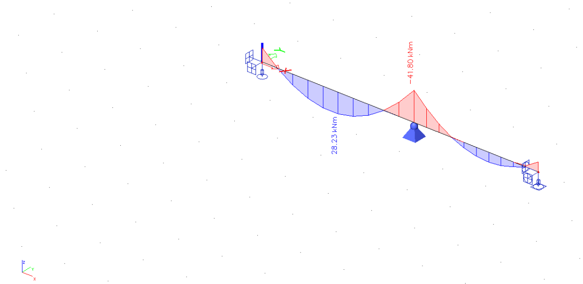
Slika 9: Momenti grede G1
