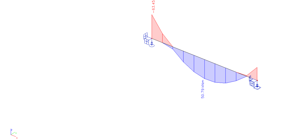
Slika 10: Momenti grede G2
