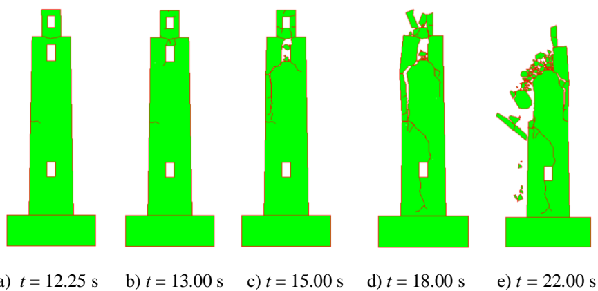
Slika 128. Širenje i nastanak pukotina za vršno ubrzanje \mathbf{a}_g = 3.30 g za Campano Lucano
