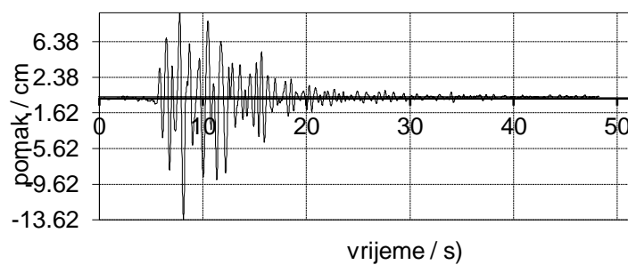
Slika 122. Vršno ubrzanje a_g = 0.46 g za Petrovac
