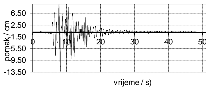
Slika 121. Vršno ubrzanje a_g = 0.45 g za Petrovac
