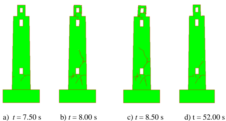
Slika 150. Širenje i nastanak pukotina za vršno ubrzanje a_g = 1.30 g za South Iceland
