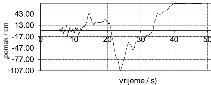
Slika 123. Vršno ubrzanje a_g = 0.48 g za Petrovac
