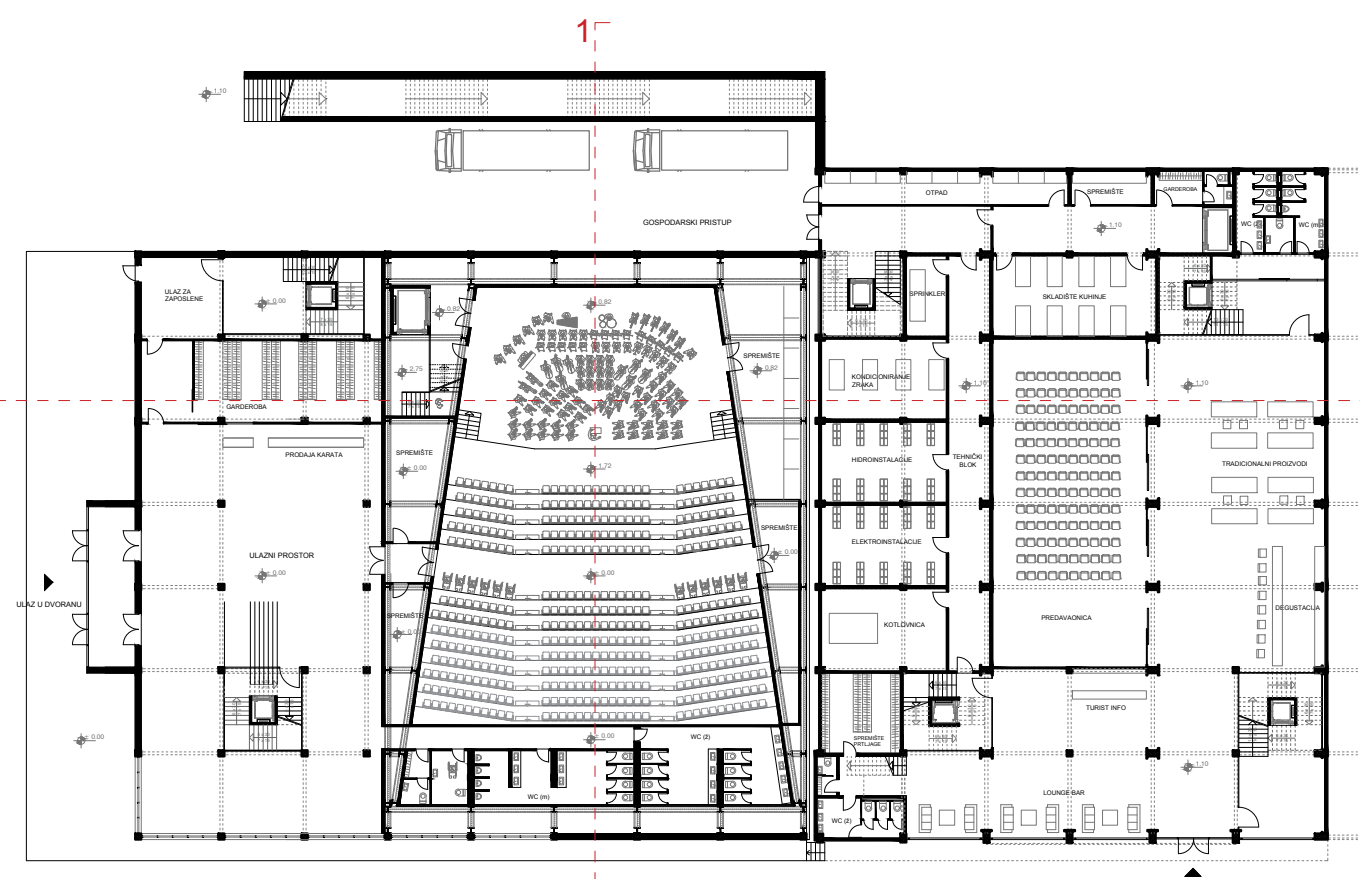
PRIZEMLJE ±0.00
