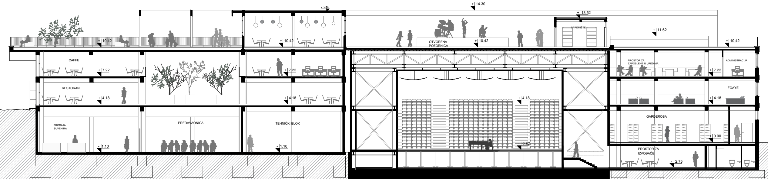
PRESJEK 2 - 2
