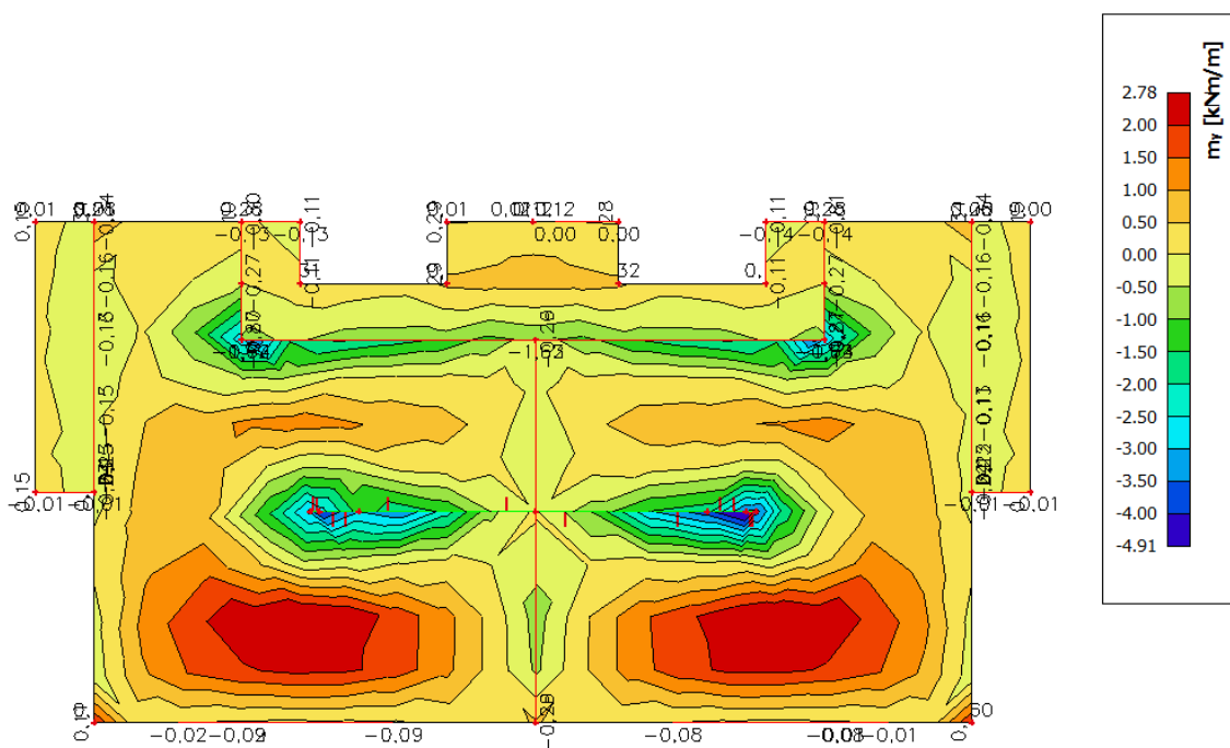
Slika 6.8 Potrebna površina armature A_s(\text{cm}^2/\text{m}) u y smjeru
