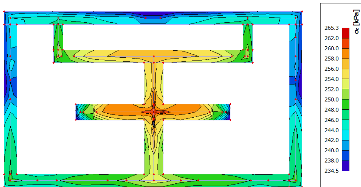
Slika 10.5 Napreznja građevine na mjestima oslanjanja temeljne stope na tlo (kPa) za kombinaciju GSN-1
