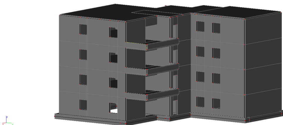
Slika 2.2 Proračunski model objekta – pogled 2
