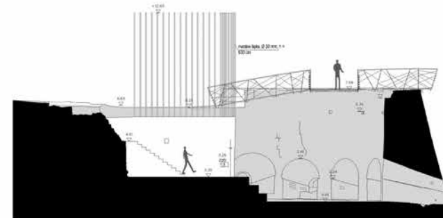
presjek 2-2
