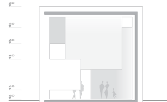
PRESJEK 1 1:100
