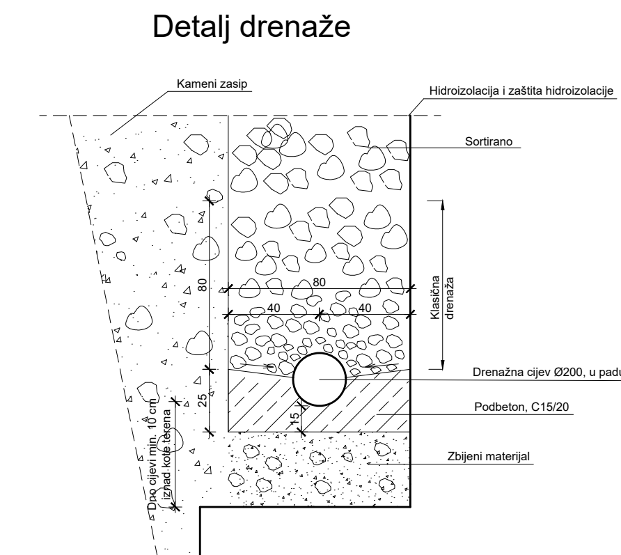
Detalj drenaze
