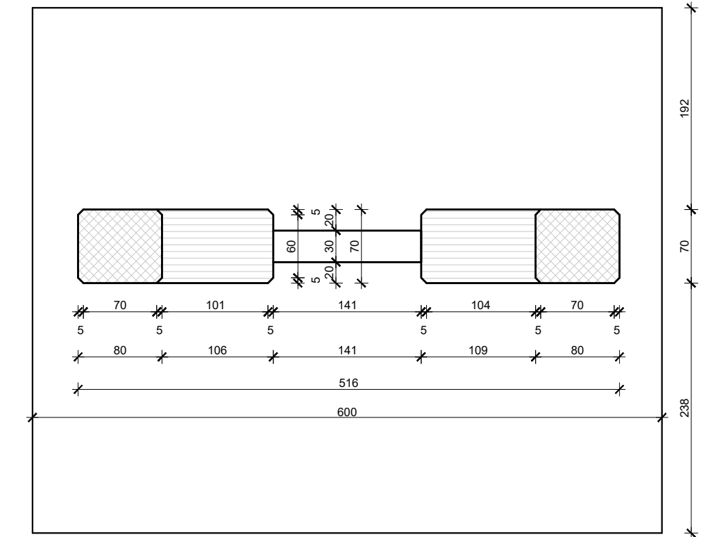
Presjek 3-3
