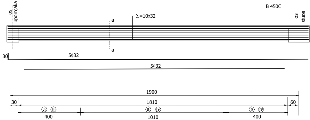
Slika 33: Uzdužni presjek nosača
