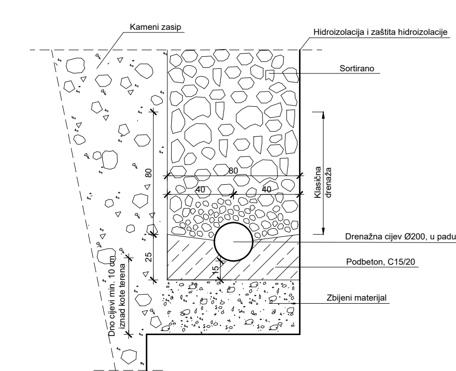
Detalj drenáže
