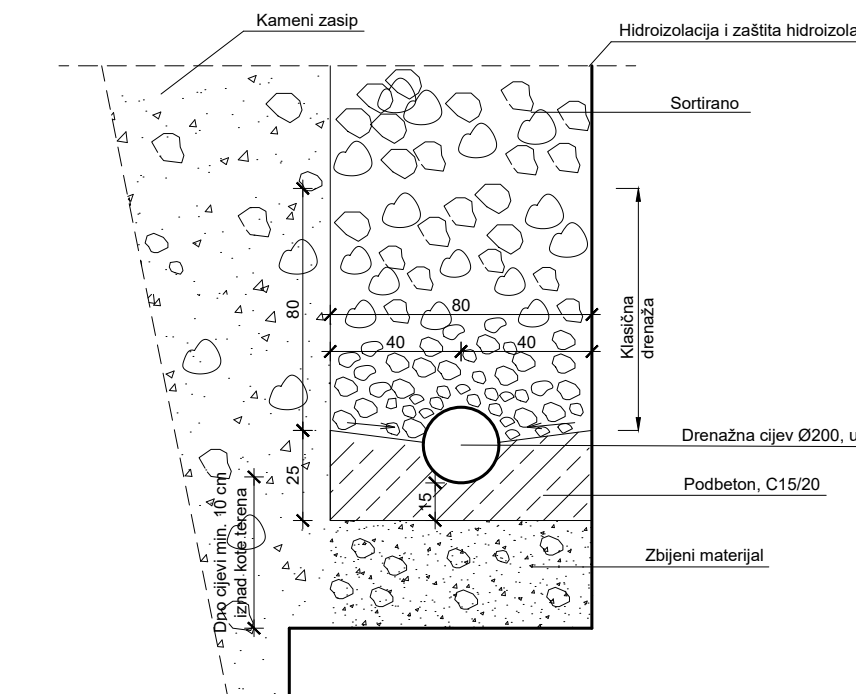
DETALJ DRENAŽE
