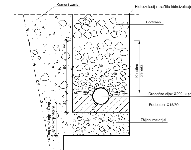
Detalj drenaže
