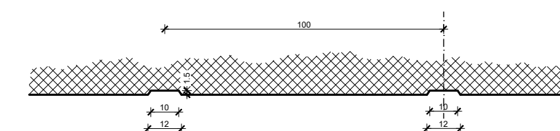
Detalj drenaže
