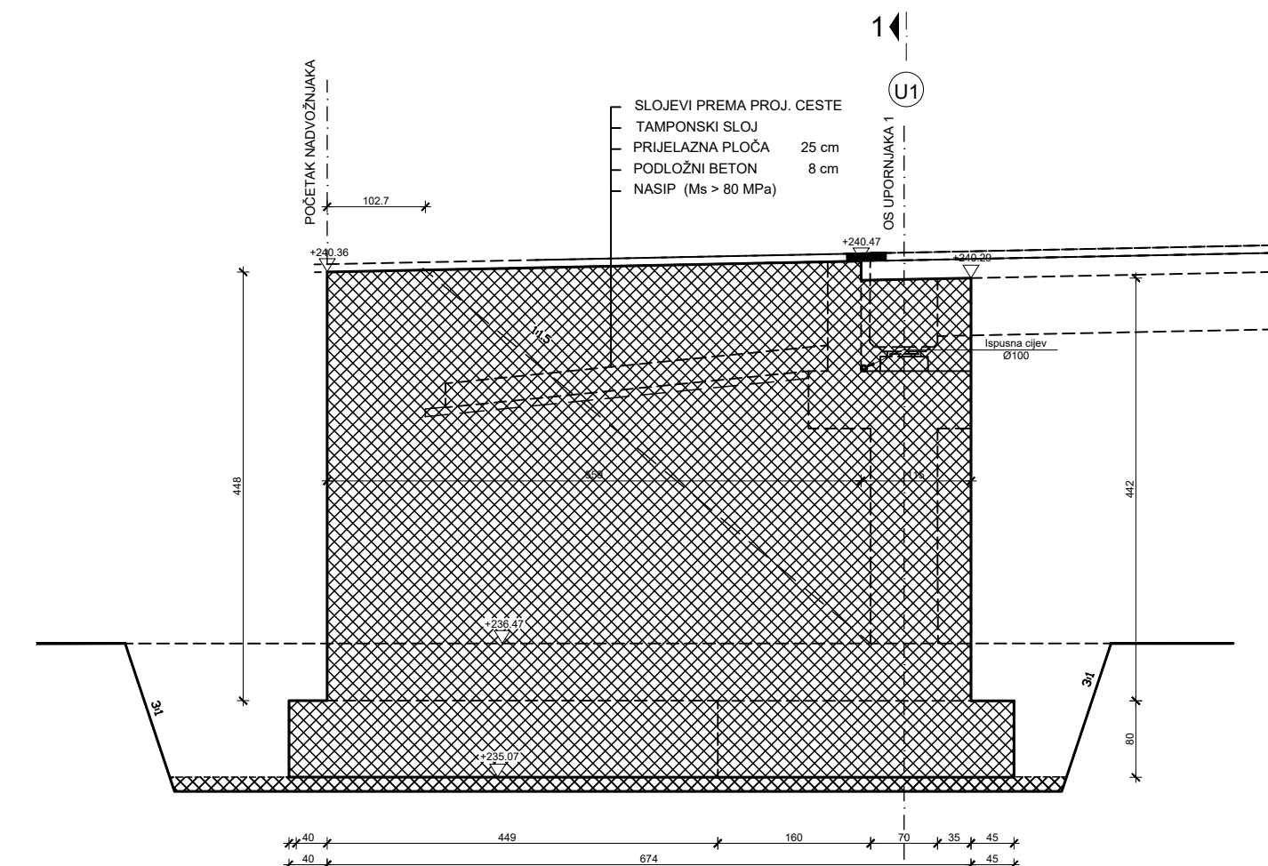
PLAN OPLATE UPORNJAKA U1 1:50
