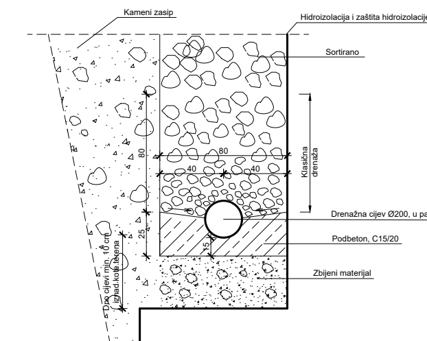
Detalj drenaže
