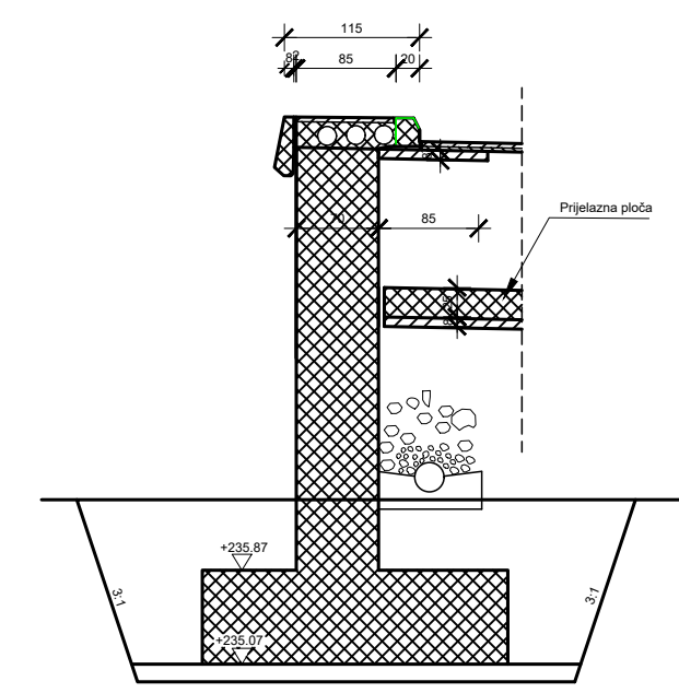
Detalj drenaže
