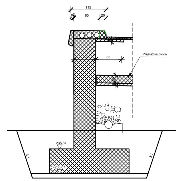
Detalj drenaže
