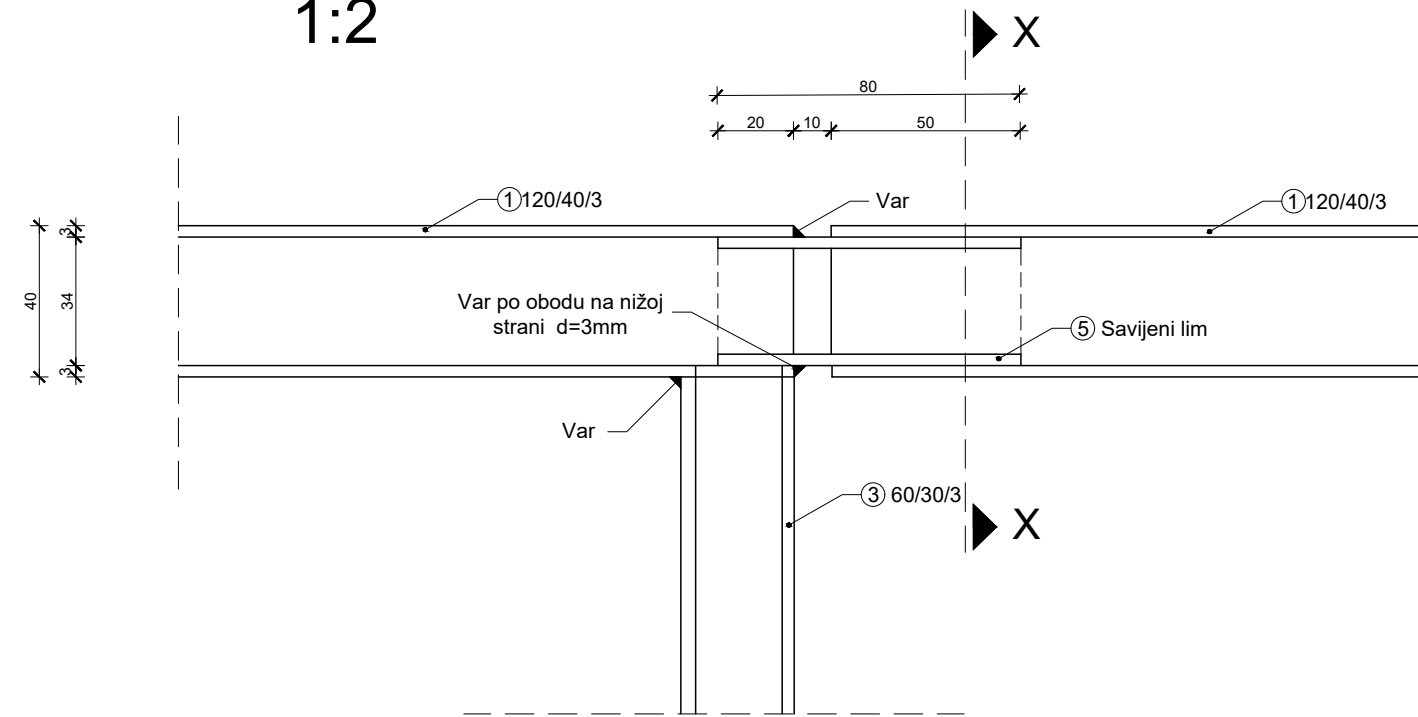
Detalj D 2 1:2
