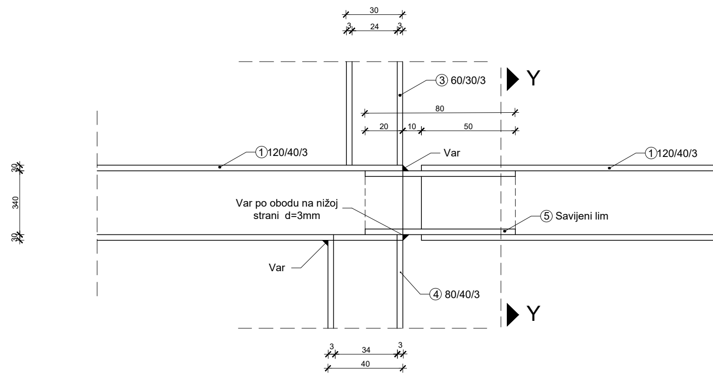
Detalj D 2 1:2
