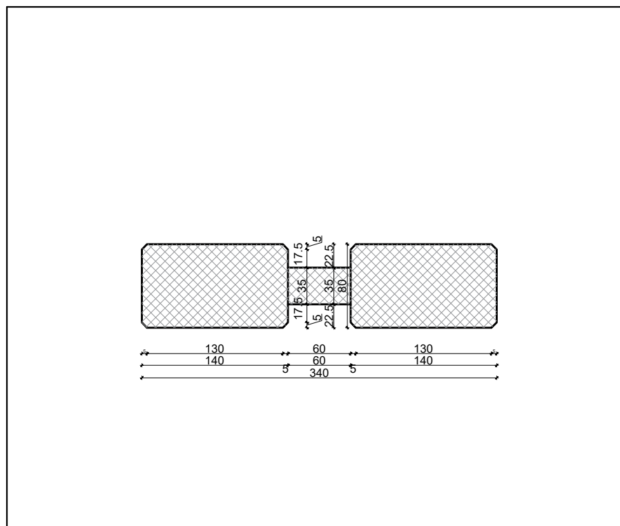
Presjek 4-4
