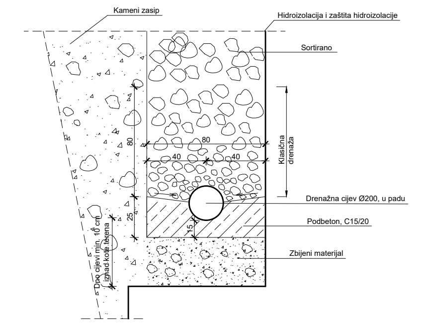
Detalj drenaže
