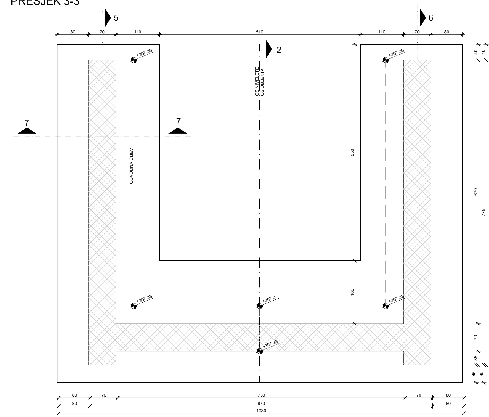
PRESJEK 3-3
