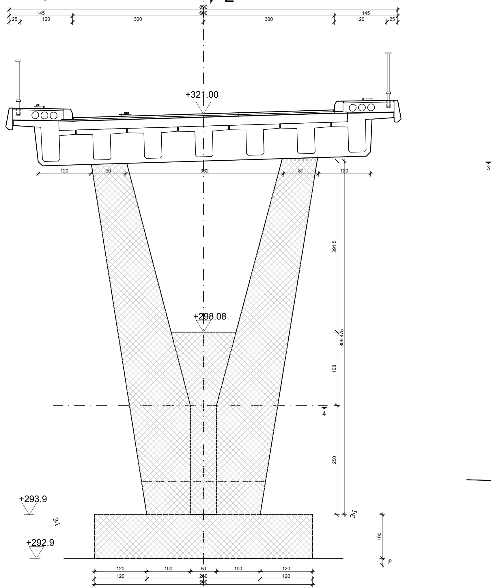
Presjek 1-1
