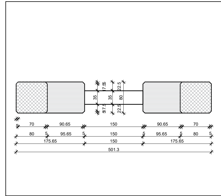
Presjek 3-3
