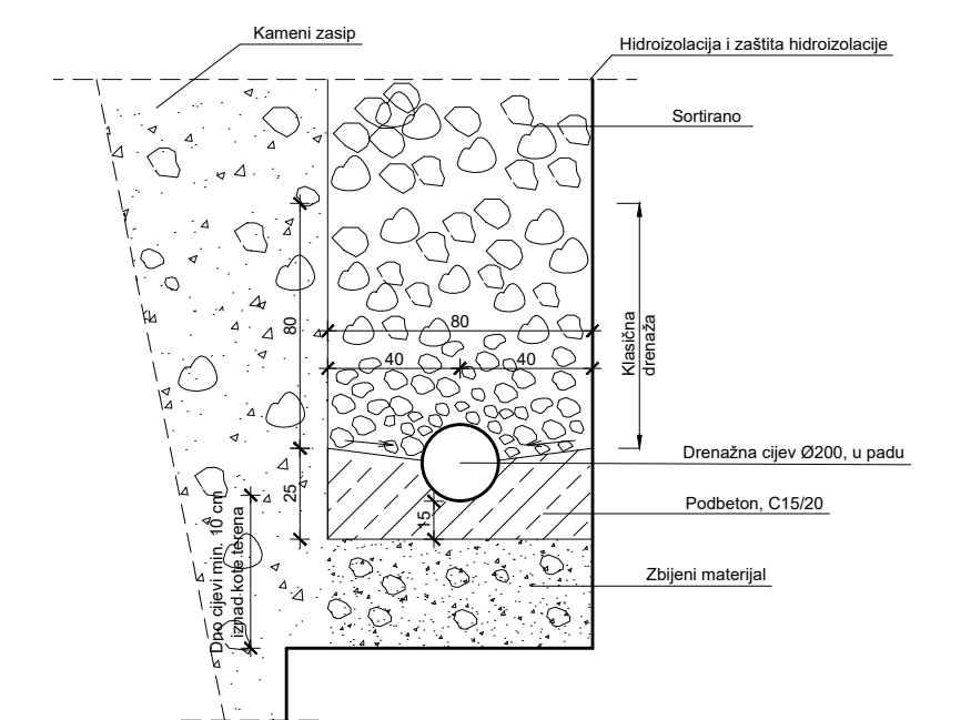
Detalj drenaze
