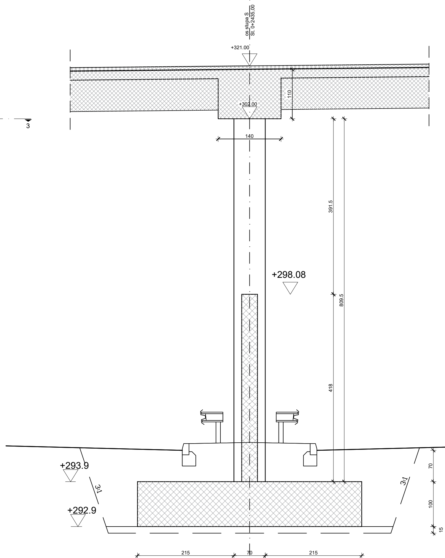
Presjek 2-2
