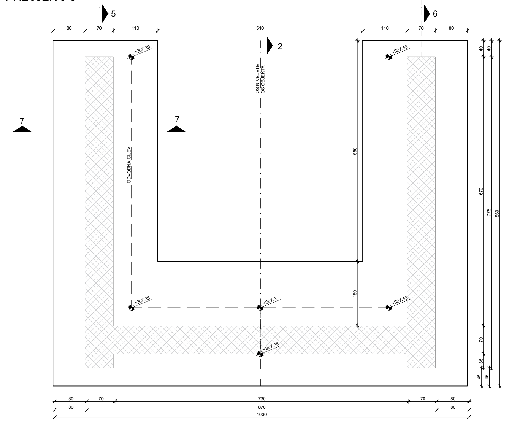
PRESJEK 3-3
