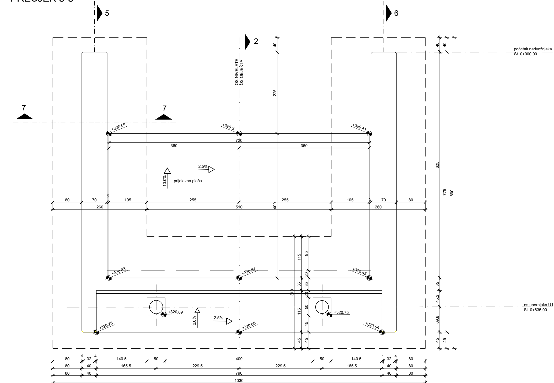
PRESJEK 3-3
