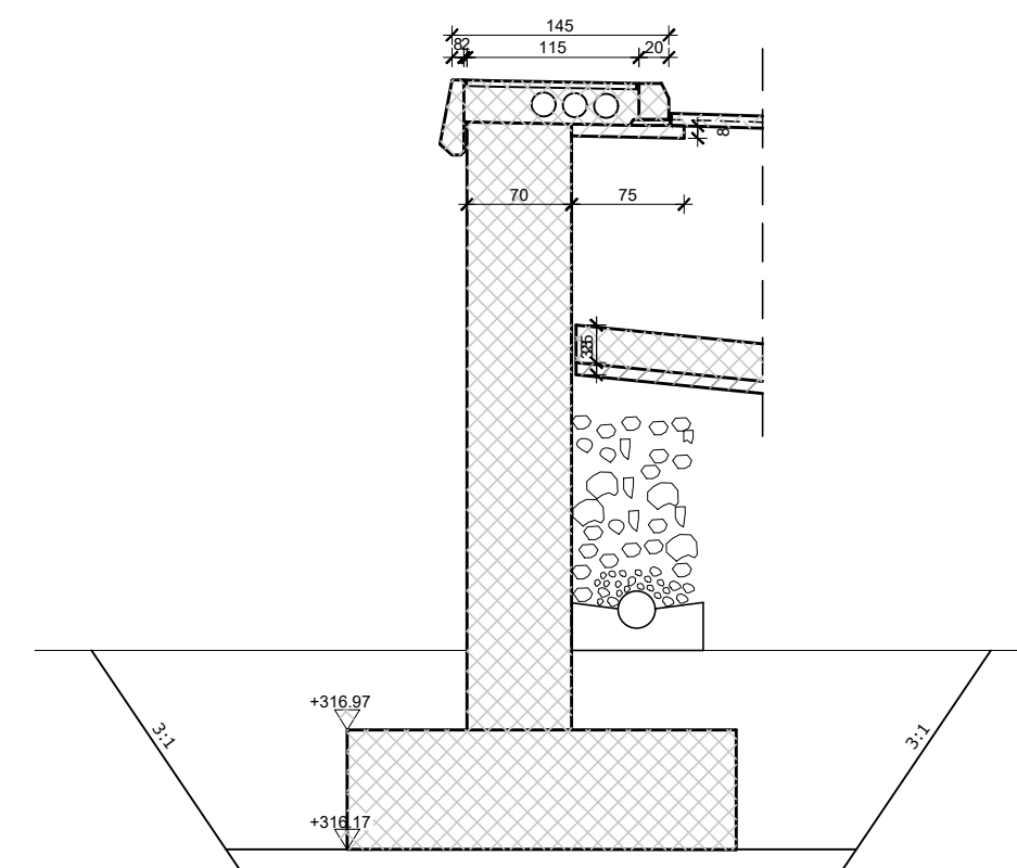
PRESJEK 7-7
