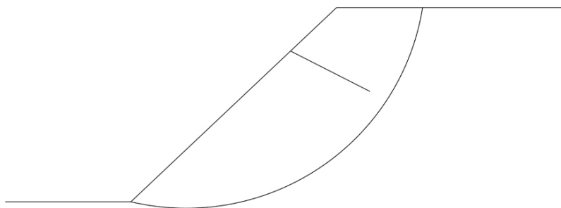
Slika 22. Sidro ne presjeca kliznu plovu [2]
