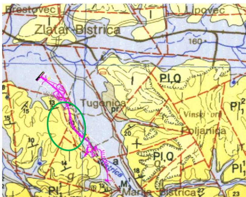
Slika 10. Izvadak iz Osnovne Geološke karte Republike Hrvatske [3]
