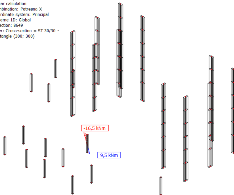
10.11 Prikaz pripadajućeg momenata savijanja M y
