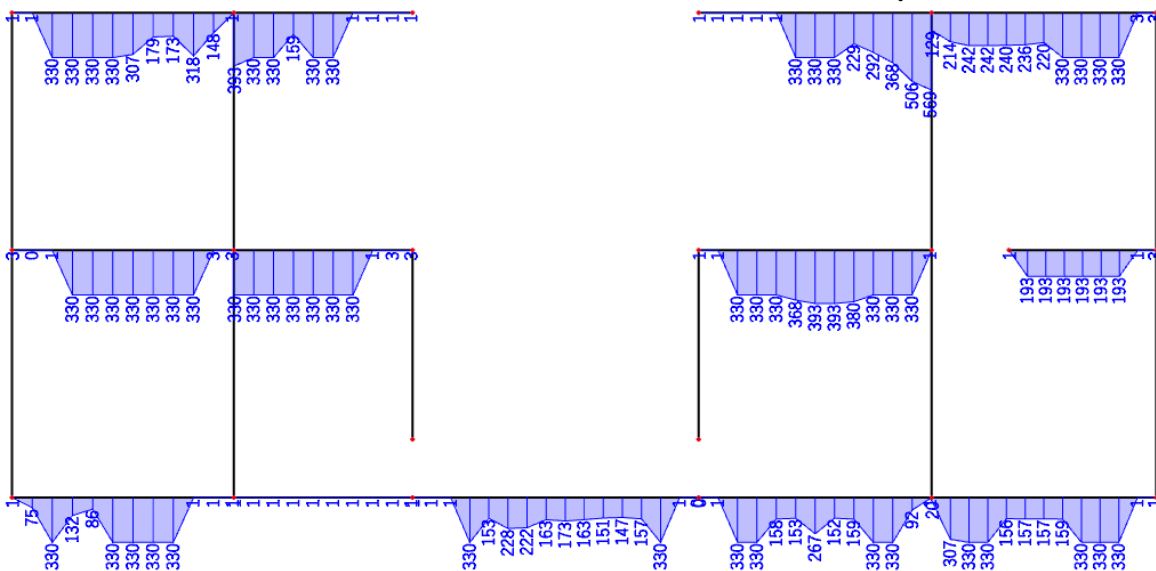
9.29 Površina potrebne armature - donja zona - X smjer
