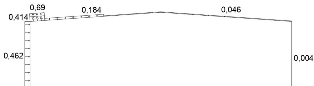
Slika 2.3.3.4. Rezultat pritiska vjetra za 2. kombinaciju
