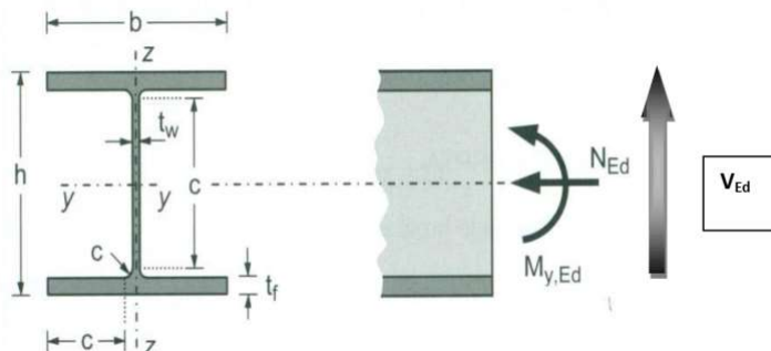
Slika 7.1.1. Skica poprečnog presjeka zabatnih stupova
