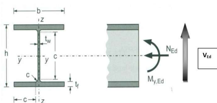
Slika 6.5.1. Skica poprečnog presjeka stupova
