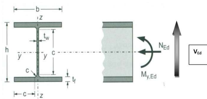
Slika 7.5.1. Skica poprečnog presjeka bočnih podrožnica
