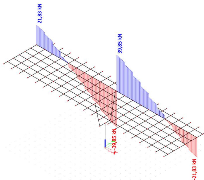
Slika 11. Dodatno stalno opterećenje – poprečne sile ( V_z ) u kN
