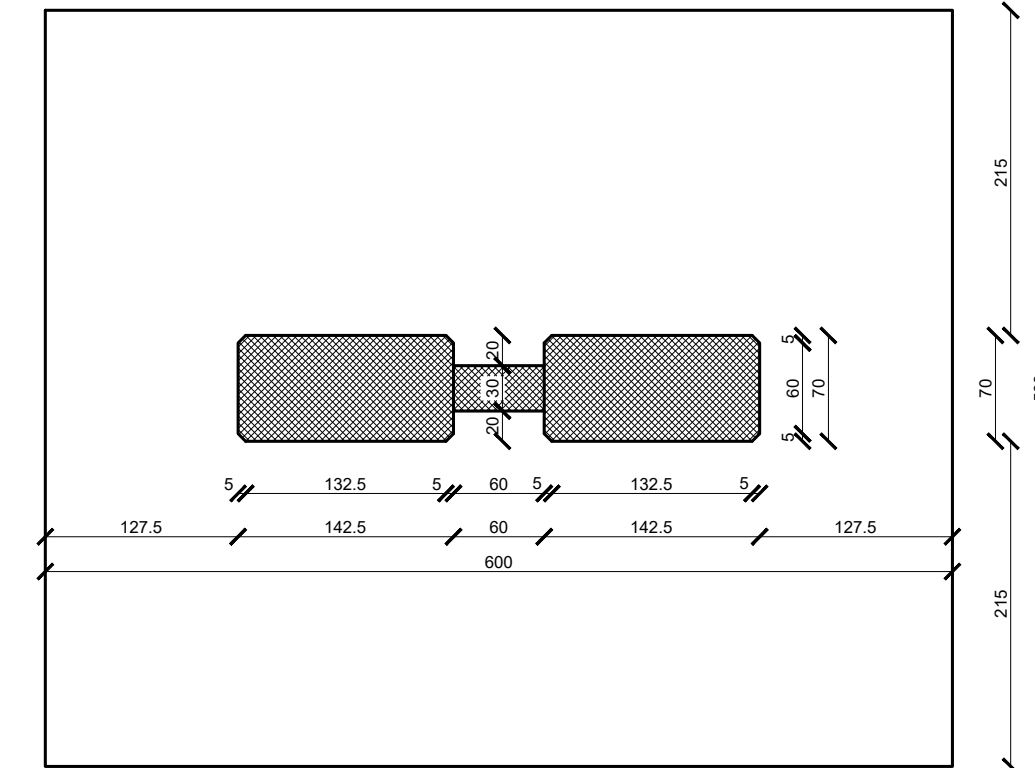
Presjek 4-4
