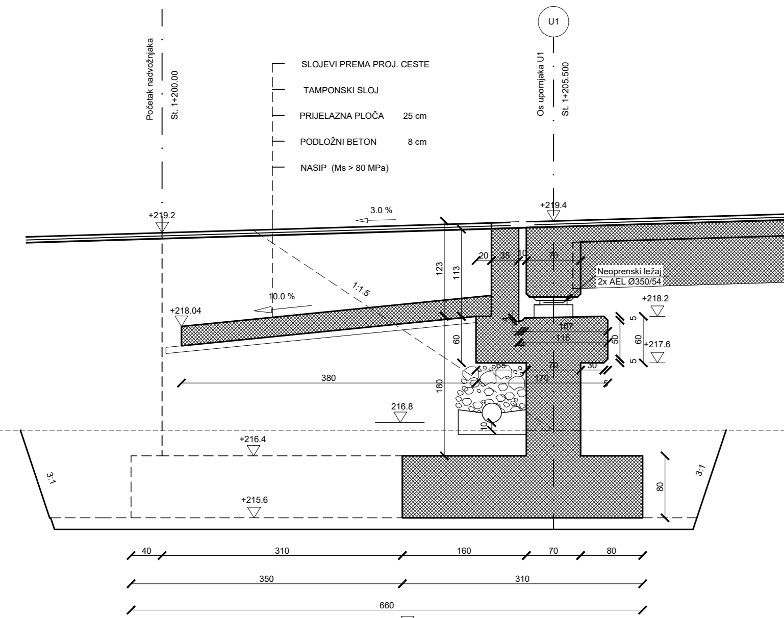
Presjek 2-2
