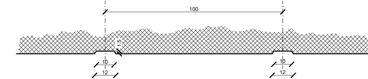
Detalj kanelura
