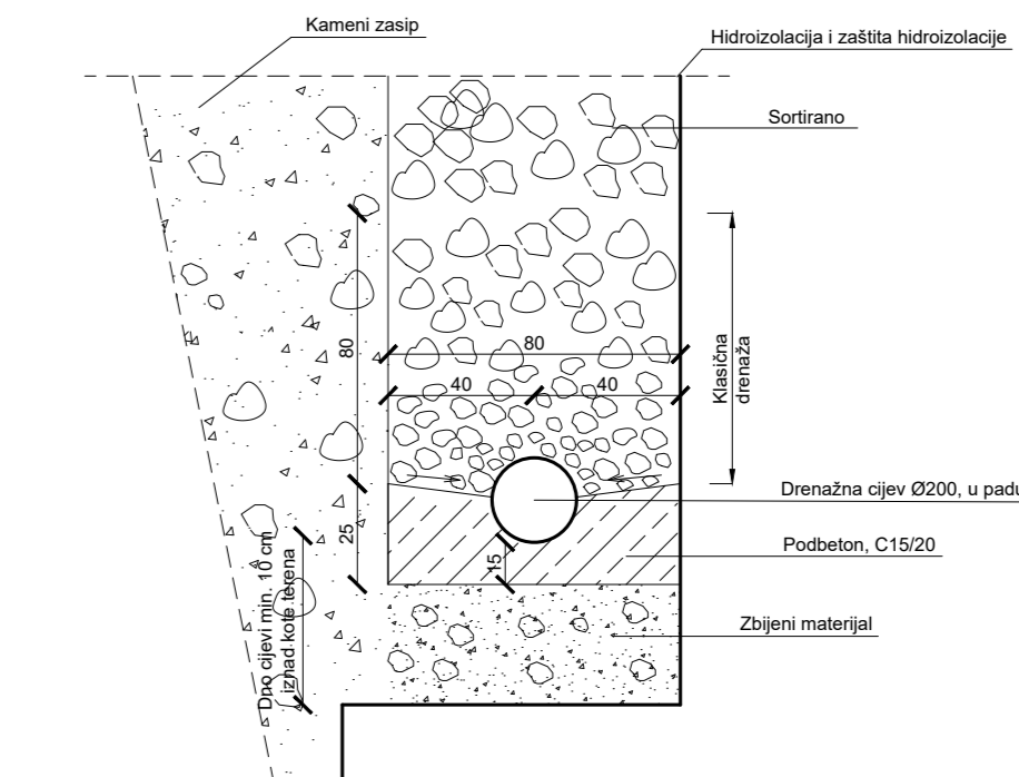
Detalj drenaže
