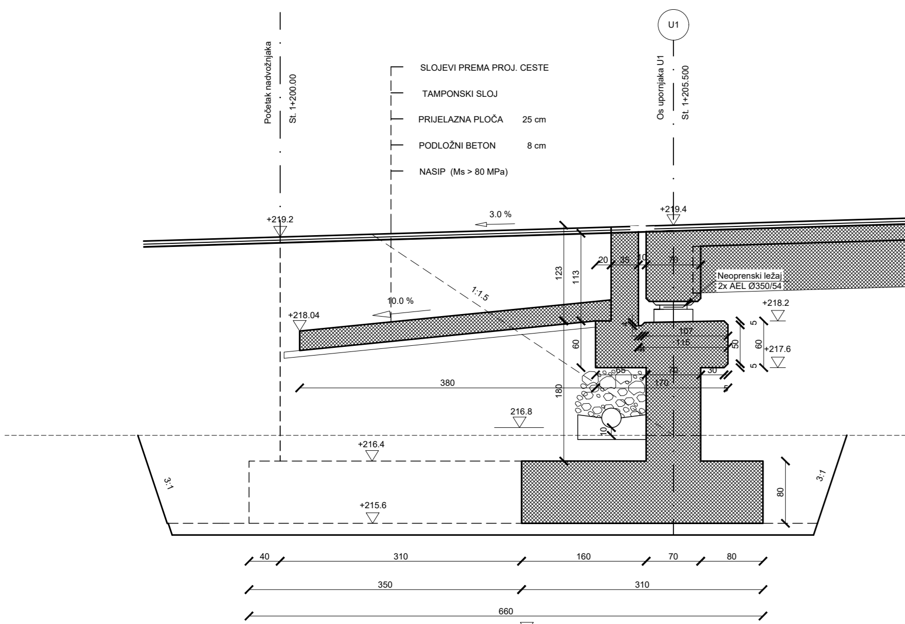
Presjek 2-2
