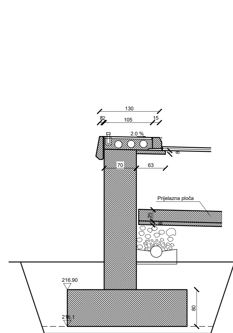
Presjek 7-7
