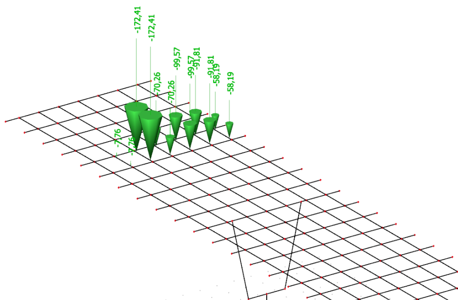
Slika 18. Prikaz opterečenja vozila za maksimalni moment nad stupom
