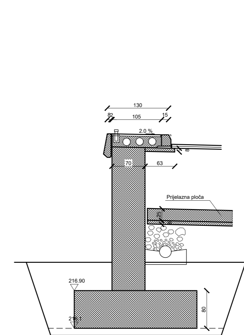
Presjek 7-7
