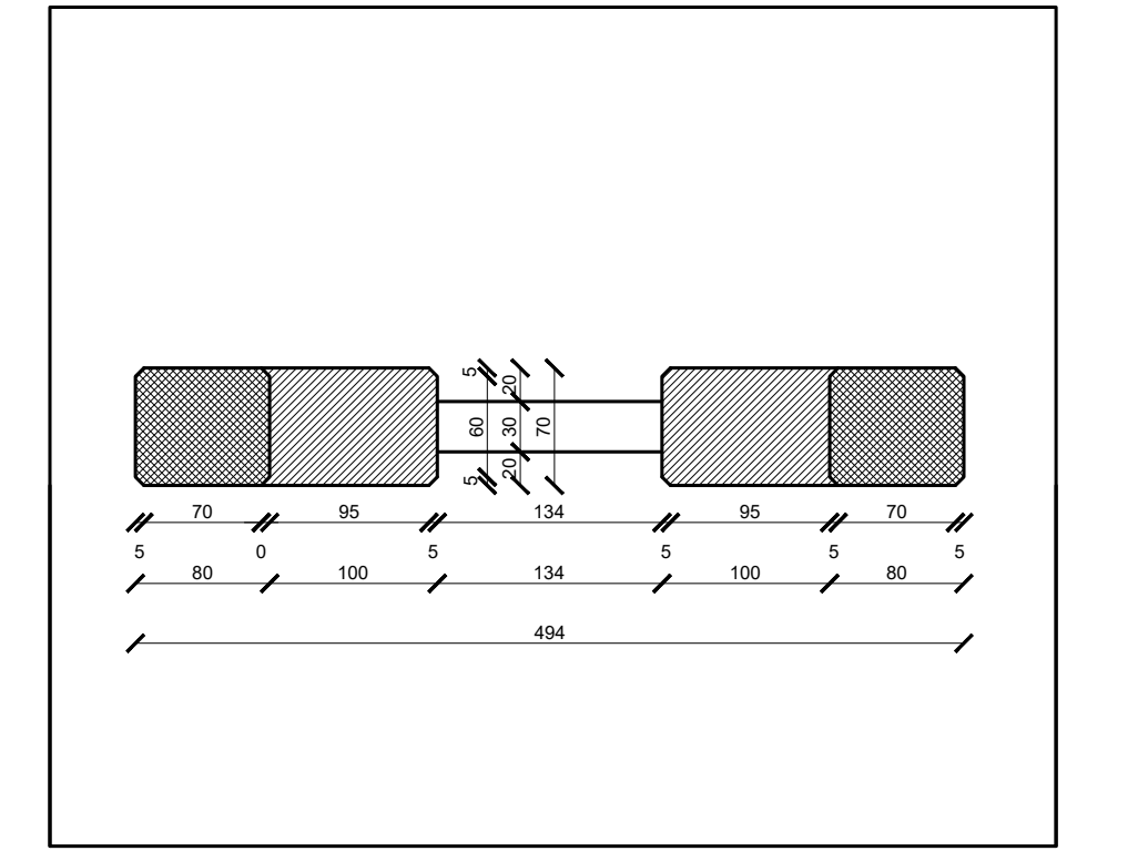
Presjek 3-3
