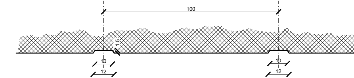
Detalj kanelura
