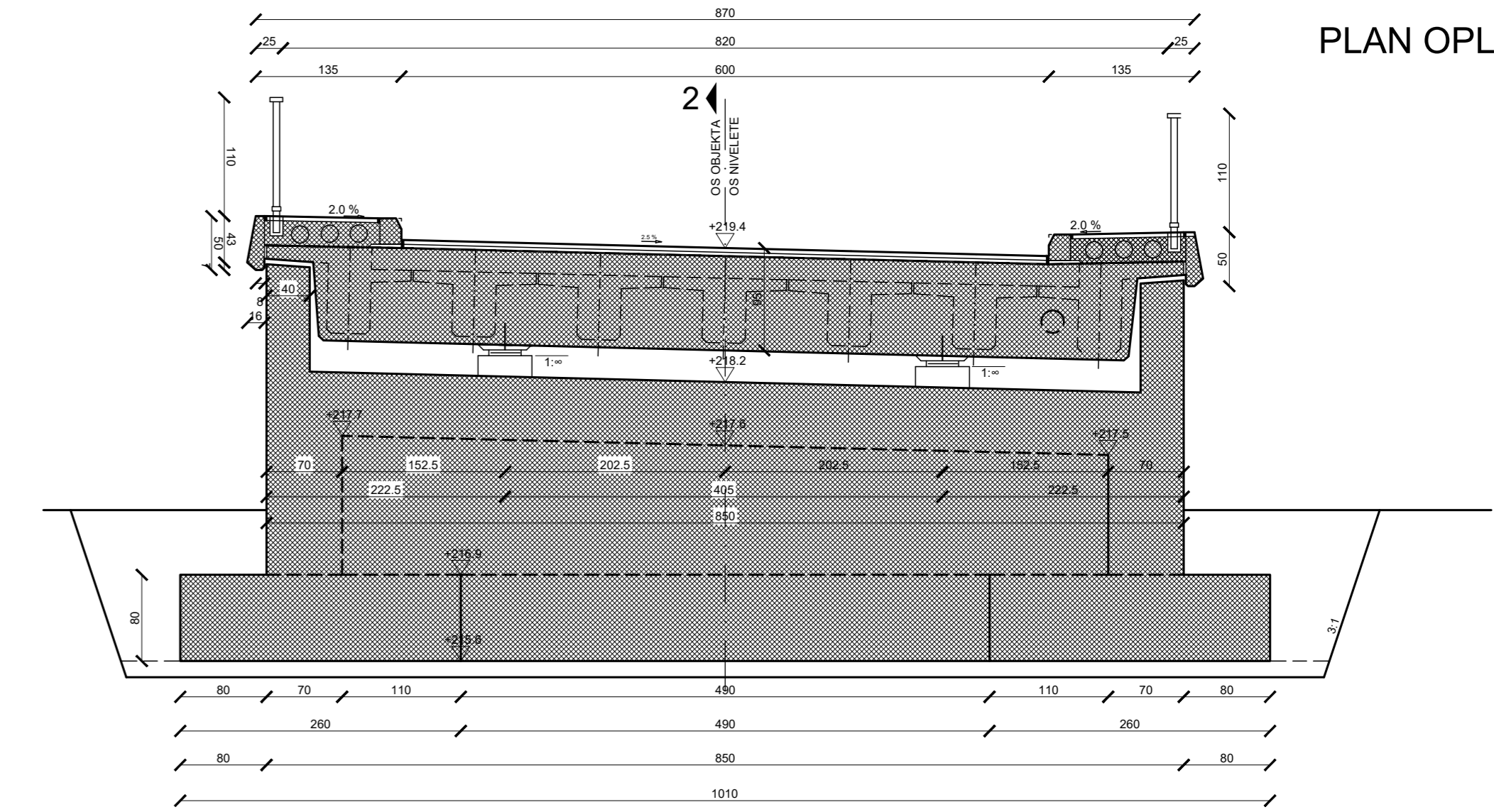
Presjek 1-1
