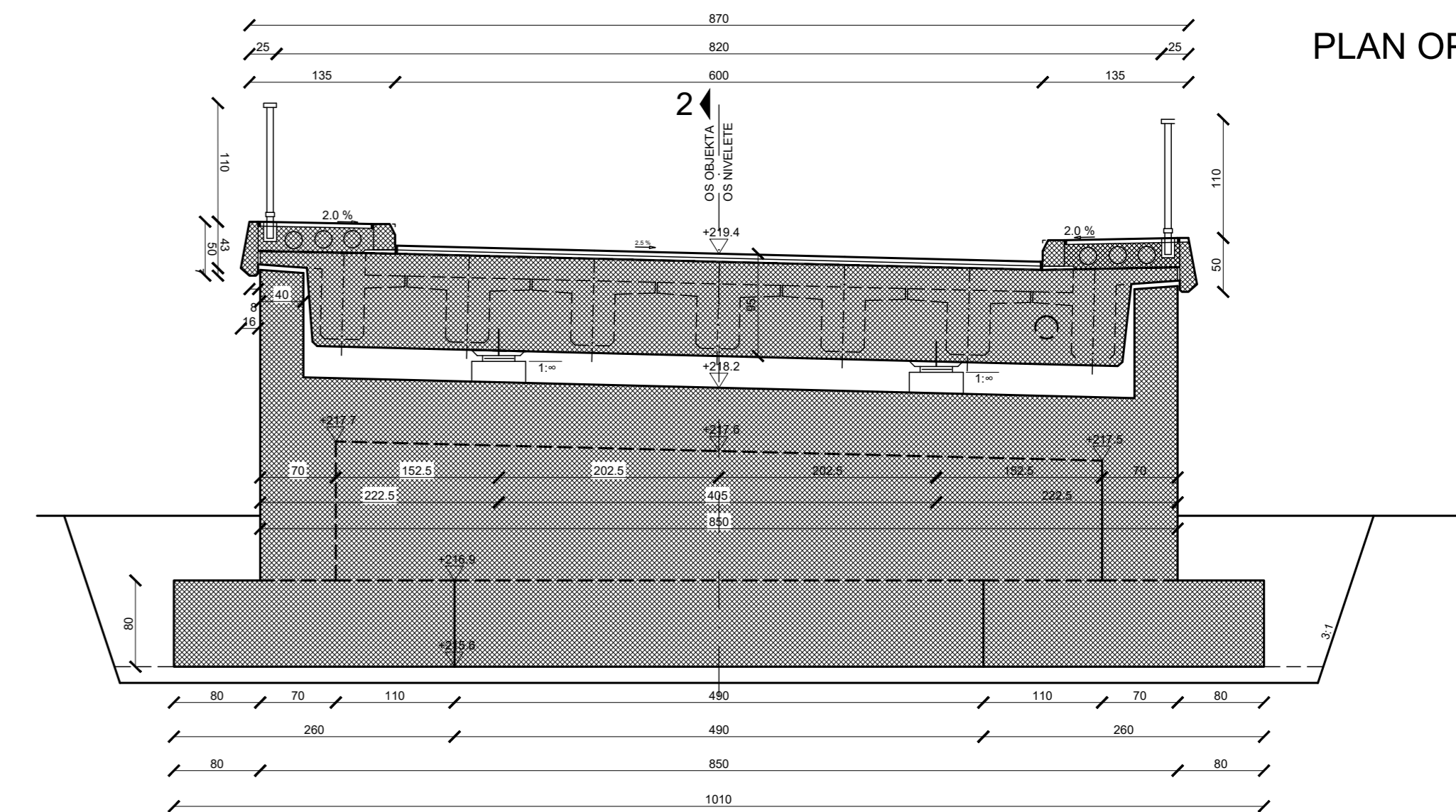
Presjek 1-1
