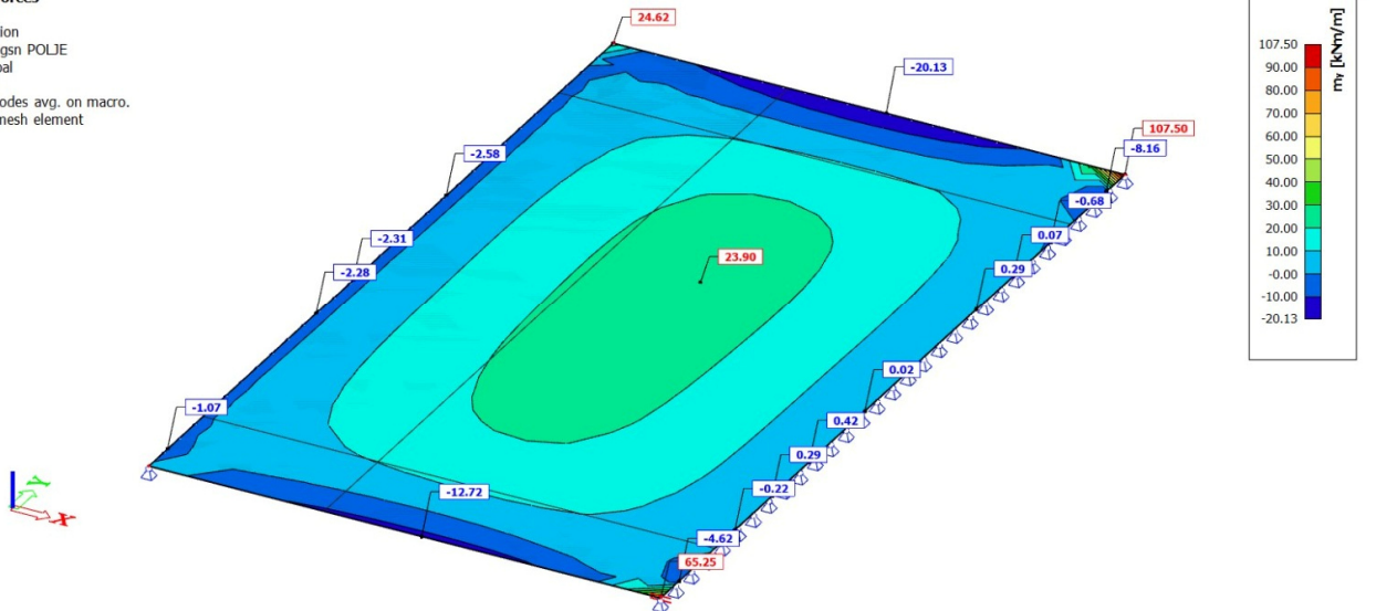
Moment m_y
