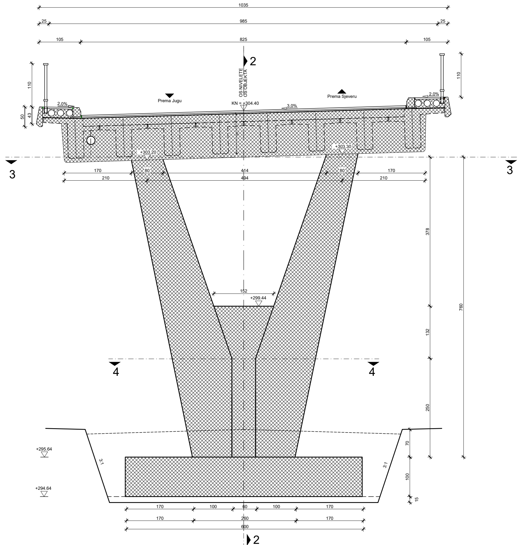
PRESJEK 1-1
