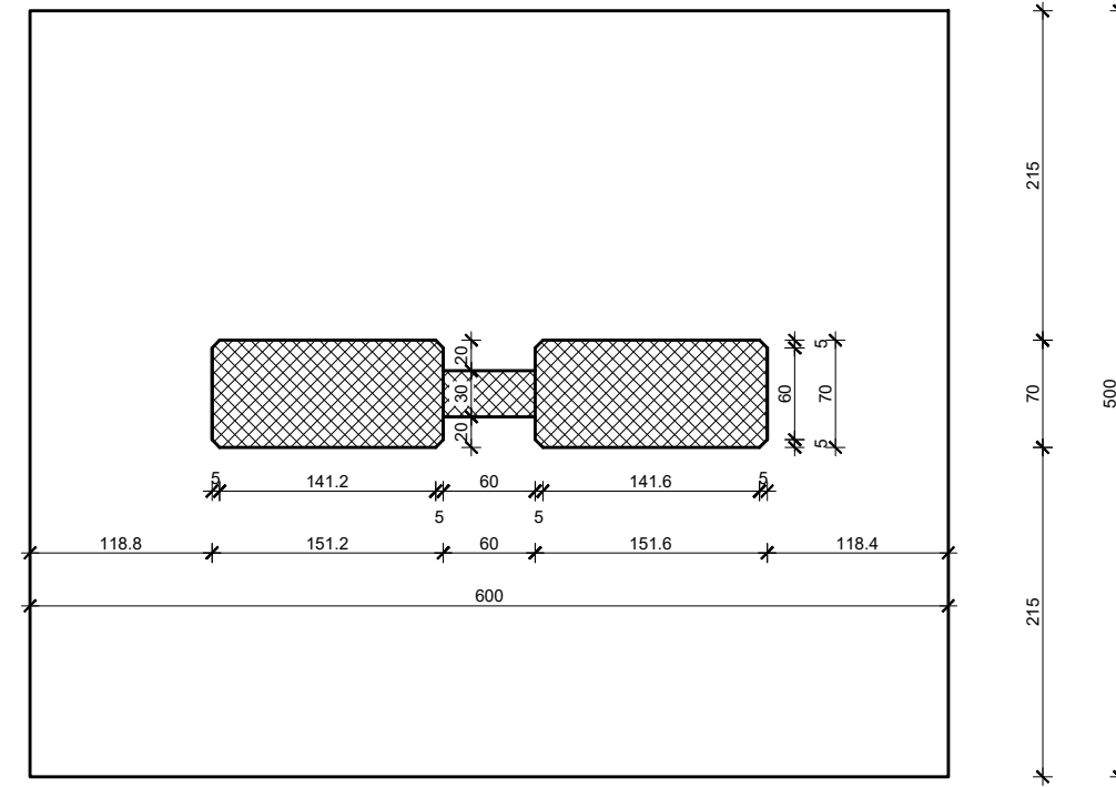
PRESJEK 4-4
