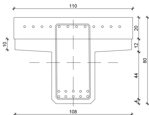
Slika 37. Dimenzije nosača
