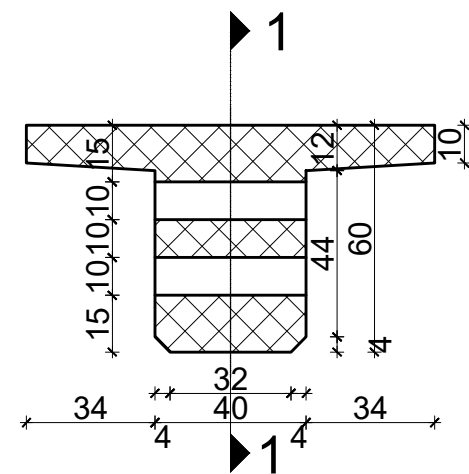
Presjek 3-3
