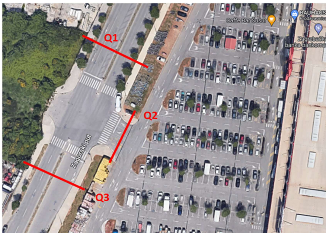
Slika 16. Nesemaforizirano raskrižje R7
