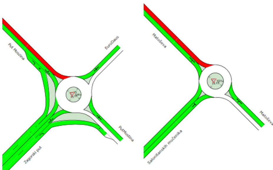
Slika 46. Vjerojatnost pojave blokiranja trakova uslijed prometne potražnje i načina rada semafora (Put Mostina – Zagorski put; Matoševa – Salonitanskih mučenika)
