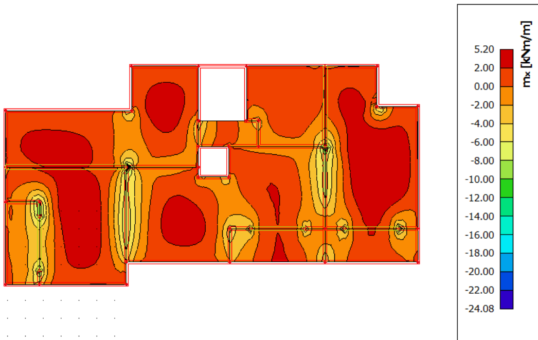
Slika 4.18. Moment savijanja M_x
