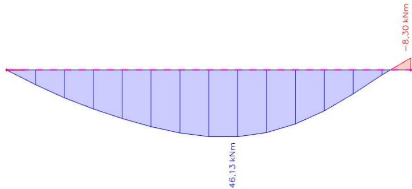
Slika 5.54. Prikaz momenata savijanja M_y od vlastite težine za gredu G 201
