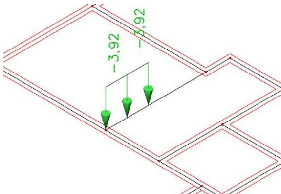
Slika 4.17. Pokretno opterećenje
