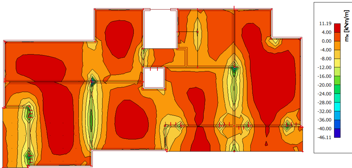
Slika 4.62. Moment savijanja M_x
