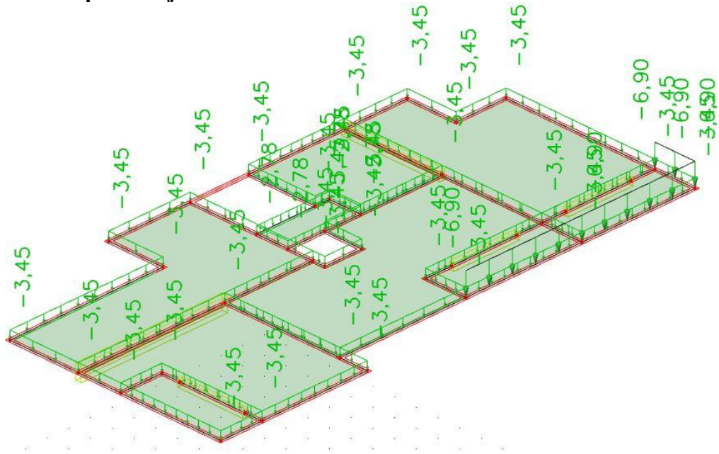
Slika 4.11. Dodatno stalno opterećenje-krov
