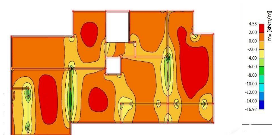
Slika 4.20. Moment savijanja M_x
