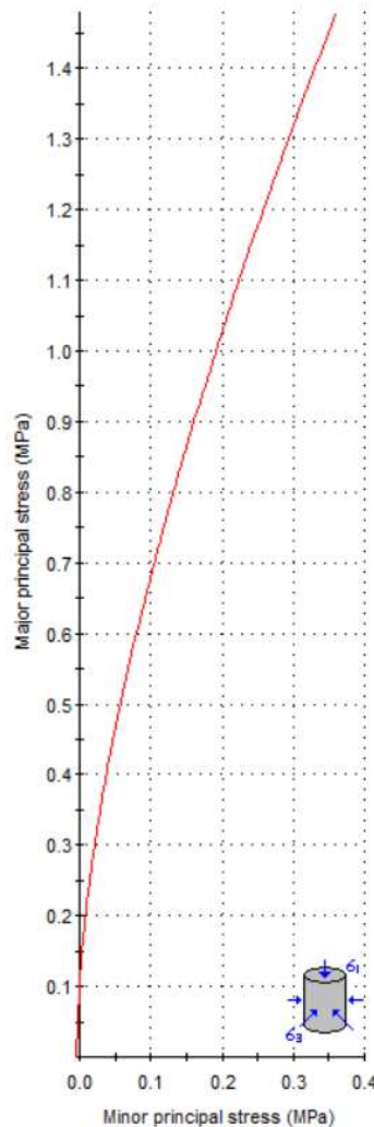
Slika 19. Dobiveni parametri u programu RocLab
