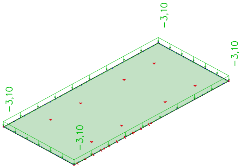
Slika 6.30. Dodatno stalno opterećenje (kN/m 2 )
