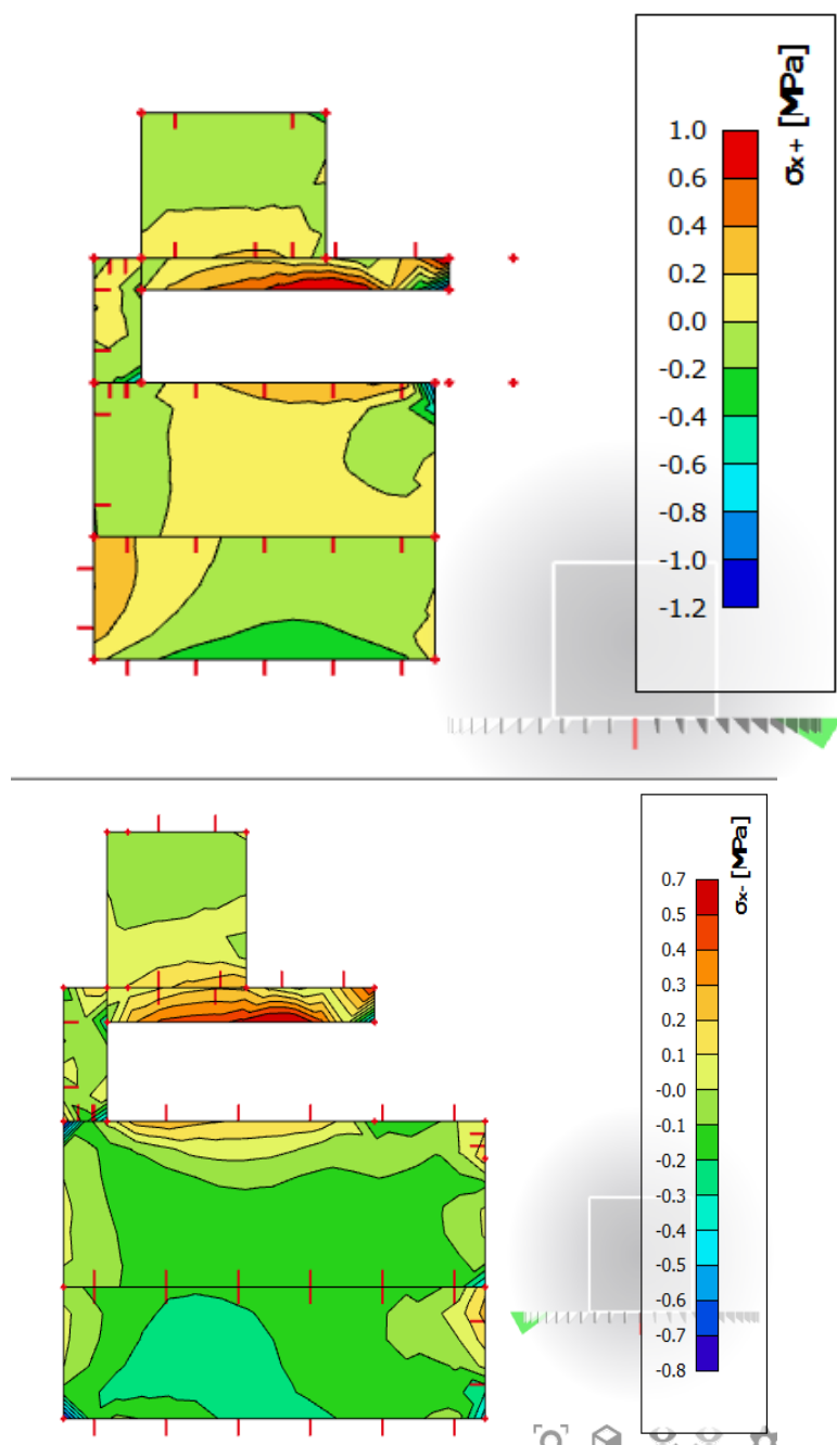
Slika 8.16. Napreznja u smjeru x
