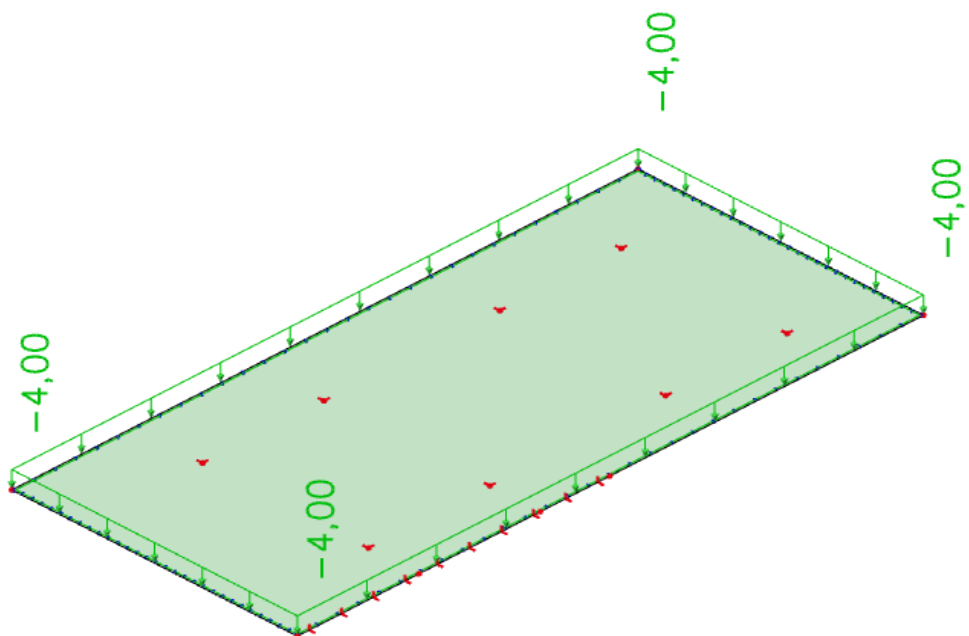
Slika 6.31. Korisno opterećenje (kN/m 2 )
