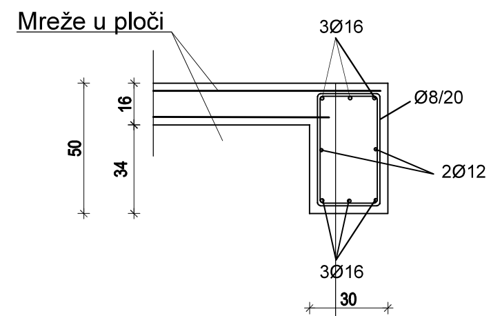
Presjek 1-1 (301)
