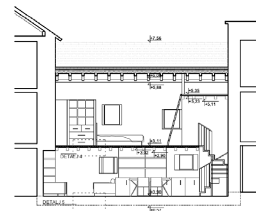
PRESJEK 3 - 3
