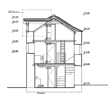
PRESJEK 2 - 2
