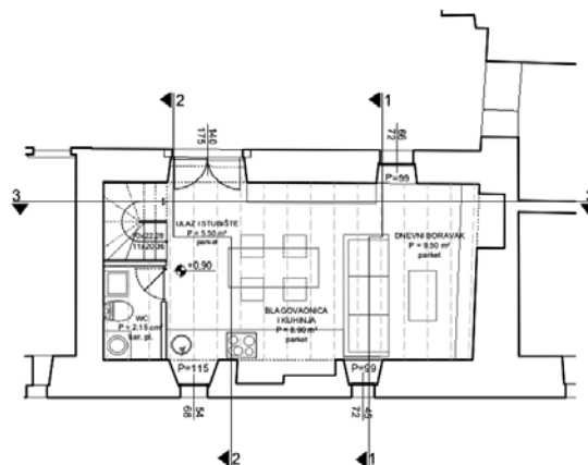
TLOCRT PRIZEMLJA
