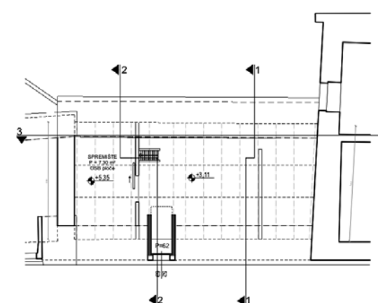
TLOCRT PODKROVLJA
