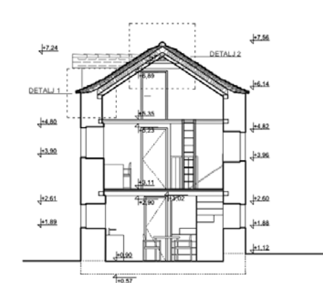
PRESJEK 1 - 1
