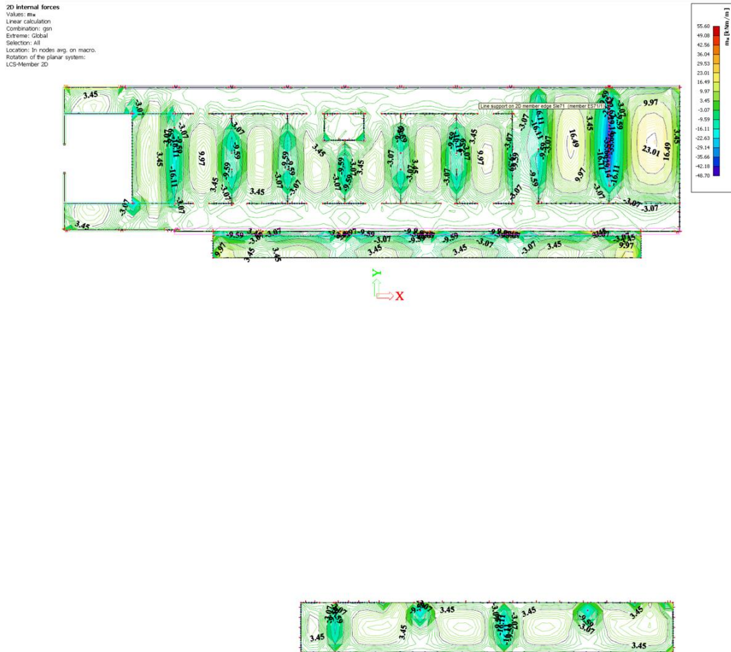
Slika 8.18. Anvelopa momenat u smjeru osi x za granično stanje nosivosti
