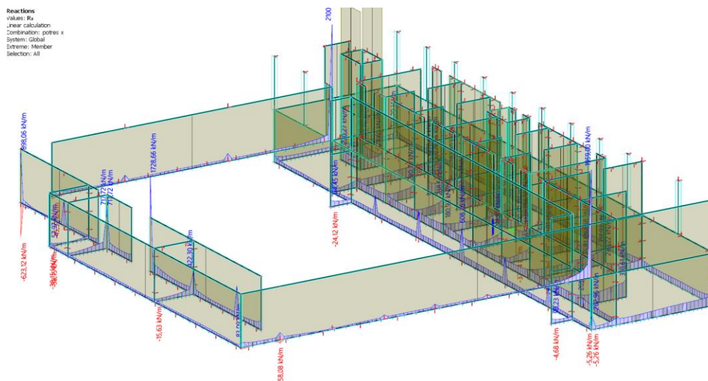
Slika 8.72. Naprezanja ispod temeljnih traka
