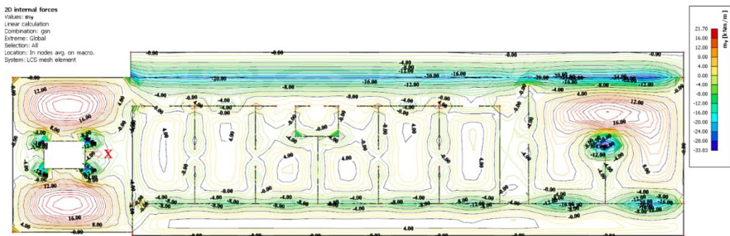
Slika 8.29. Anvelopa momenata u smjeru osi y za granično stanje nosivosti
