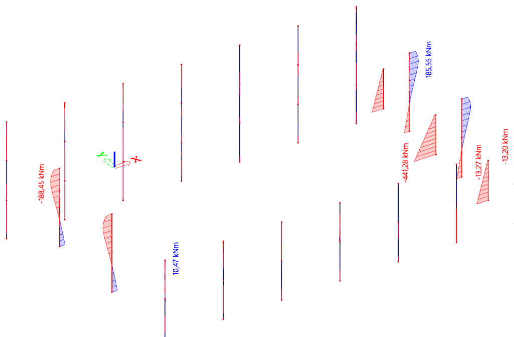
Slika 8.41. Moment savijanja oko y osi (Uobičajna kombinacija smjer x) [kNm]
