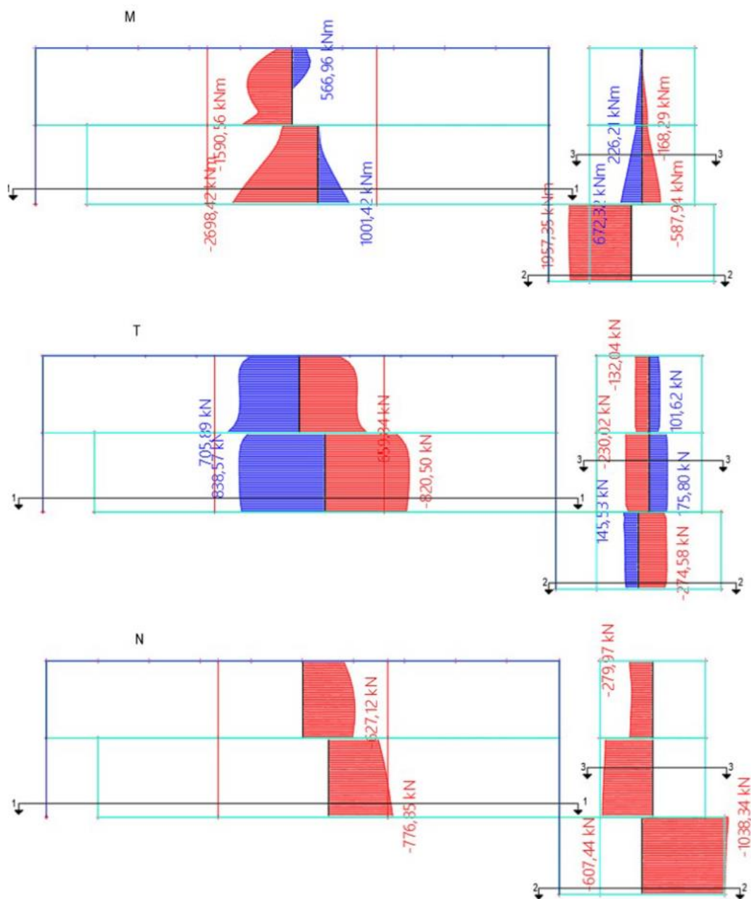
Slika 8.62. Prikaz rezultata u zidu u osi 2
