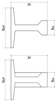
PRESJEK 1-1: PRESJEK 2-2:
