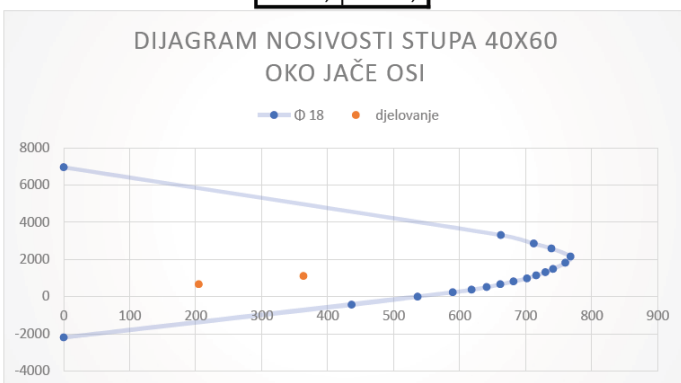
Slika 8.46. Dijagram interakcije za Φ 18
