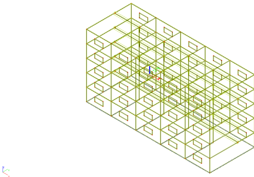
Žičani model konstrukcije (poprečni presjeci su označeni raznim bojama)
