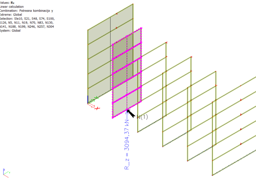
Reakcija Rz ispod promatranog zida za Potresnu kombinaciju y
