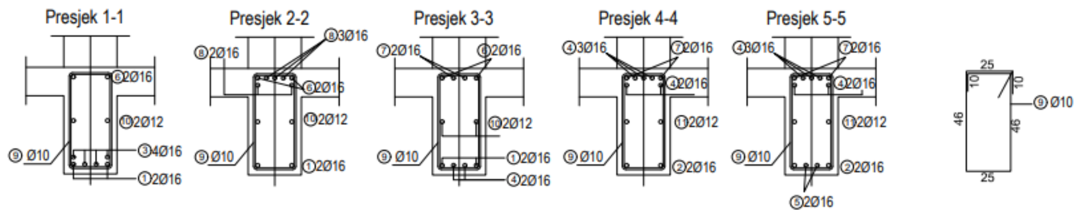
REBRASTA ARMATURA B500B
