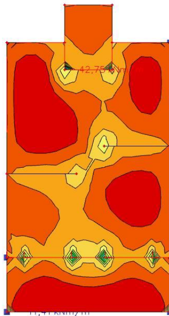
Slika 4.4. M_{Sd,x} ( kN/m^2 ) = računski momenti savijanja u smjeru lokalnih osi za q_{sd} = 1.35G + 1.5Q
