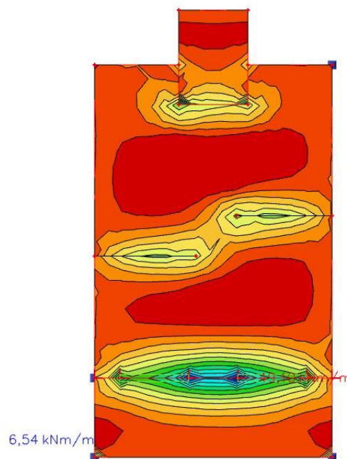
Slika 4.5. M_{Sd,y} ( kN/m^2 ) = računski momenti savijanja u smjeru lokalnih osi za q_{sd} = 1.35G + 1.5Q
