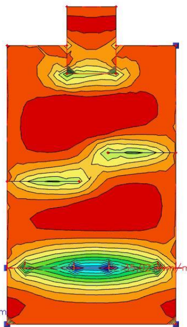
Slika 4.7. M_{Sd,y} (kN/m 2 ) = računski momenti savijanja u smjeru lokalnih osi za q_{sd} = 1.0G+1.0Q
