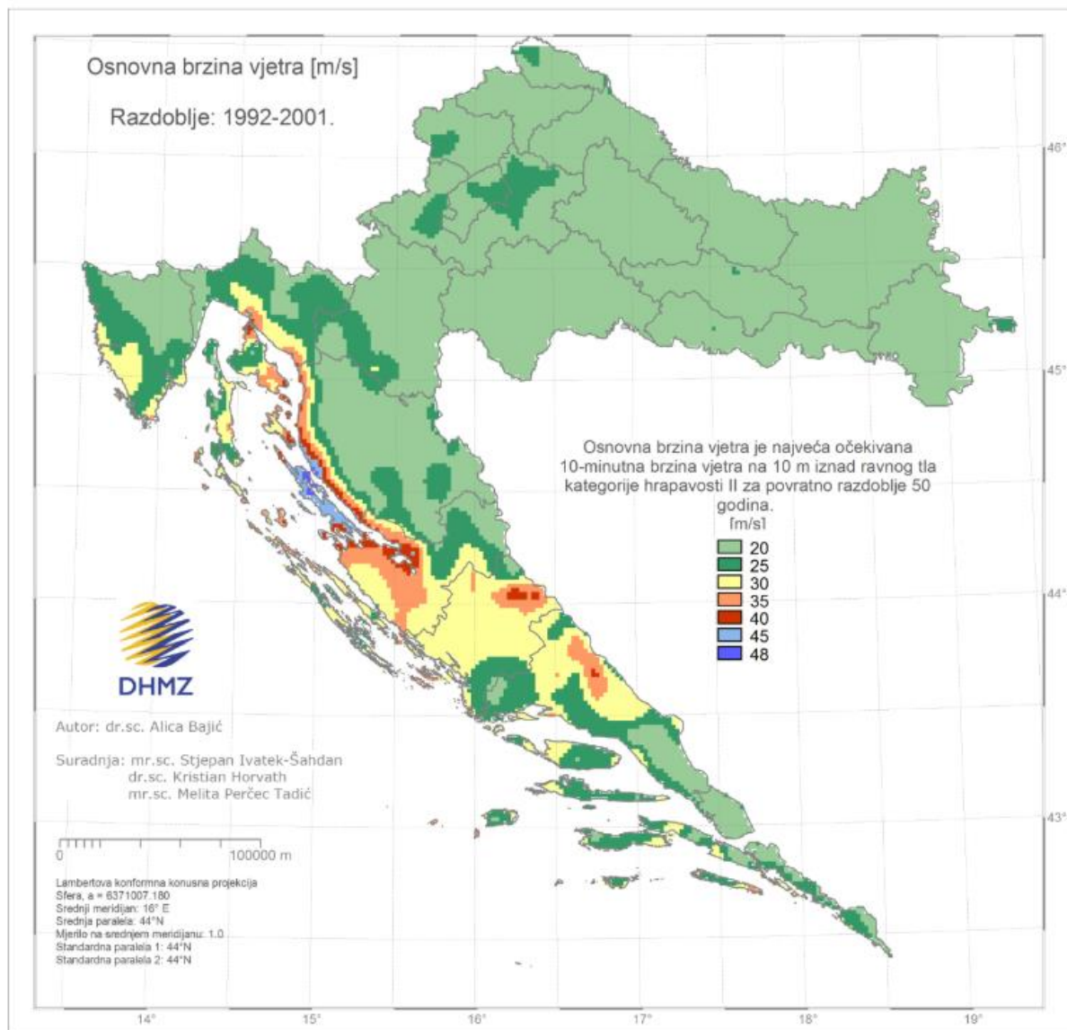
Slika 3.2. Karta osnovne brzine vjetra za RH
