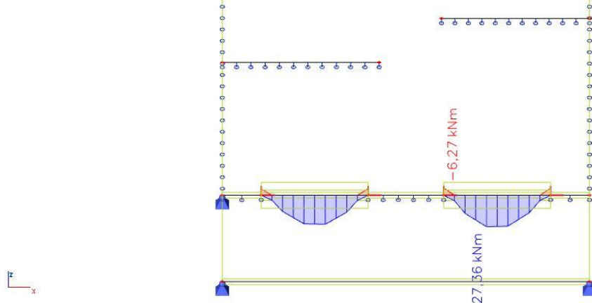
Slika 4.25. M_{sd,y} ( kN/m^2 ) = računski momenti savijanja u smjeru lokalnih osi za q_{sd} = 1.35G + 1.5Q
