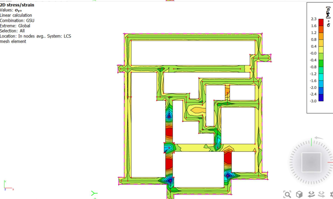
Dijagram 40.. Prikaz maksimalnih naprezanja u temeljima za kombinaciju opterećenja GSU
