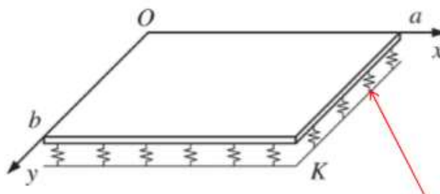
Slika 33. Međudjelovanje konstrukcija – tlo modelirano Winkler- ovim modelom
