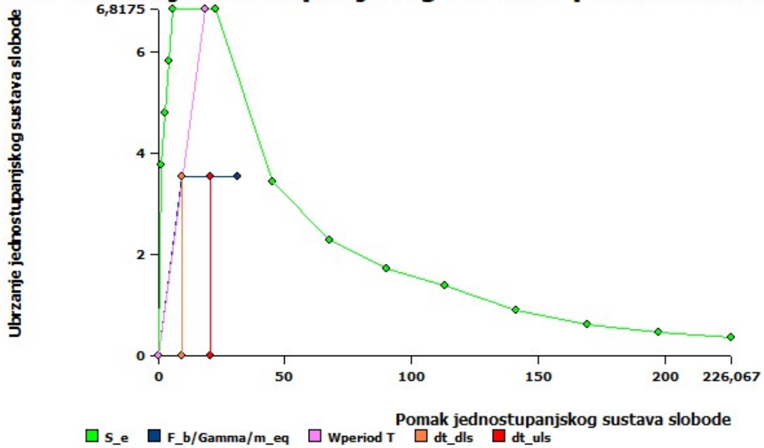
Dijagram 52. Spektar odziva jednostupanjskog sustava
