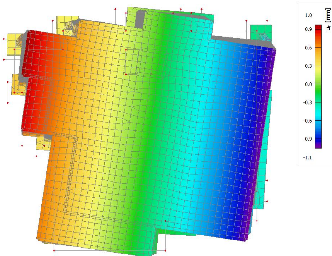
Slika 6.1.4. Prikaz rotacije građevine oko osi z
