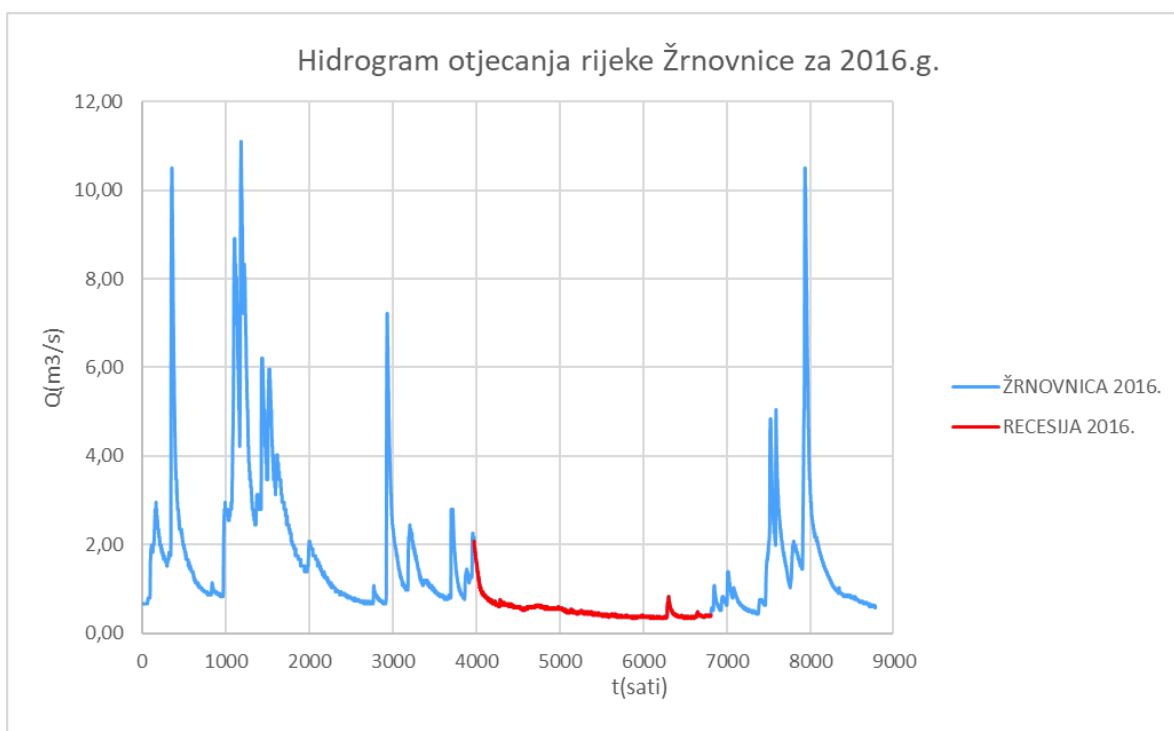
Slika 36. Hidrogram otjecanja i recesija rijeke Žrnovnice za 2016. godinu
