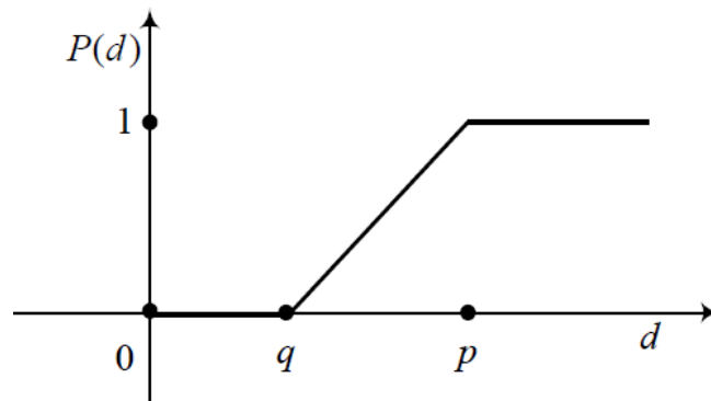
Slika 19.- graf funkcije preferencije s linearnom preferencijom i područjem indiferencije
