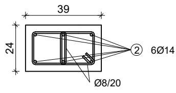
DETALJ ⑧
